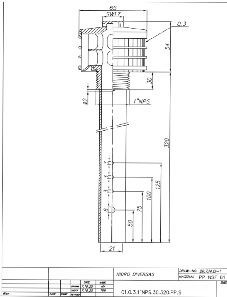
Dibujo de Ingeniería boquilla para filtros planta Picacho SANAA
