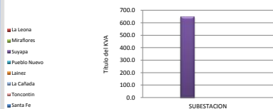
DEMANDA PROYECTADA POR DISEÑOS EN 13.8 KV
