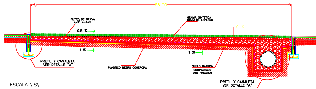
SECCION LONGITUDINAL DE CANCHA
