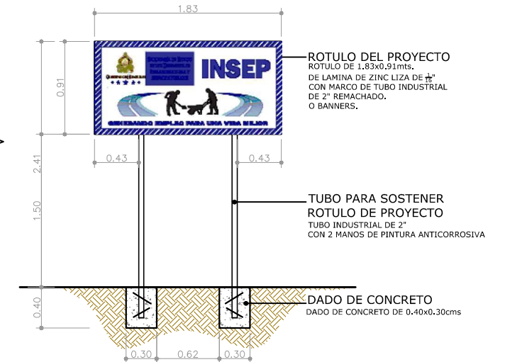
DETALLE DE ROTULO DEL PROYECTO ESCALA: S/E
