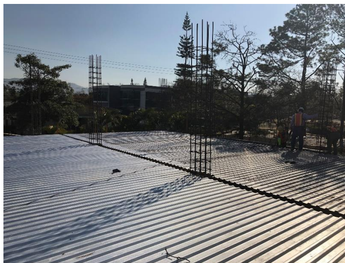
Imagen 7. Armado de Losa de Entrepiso
