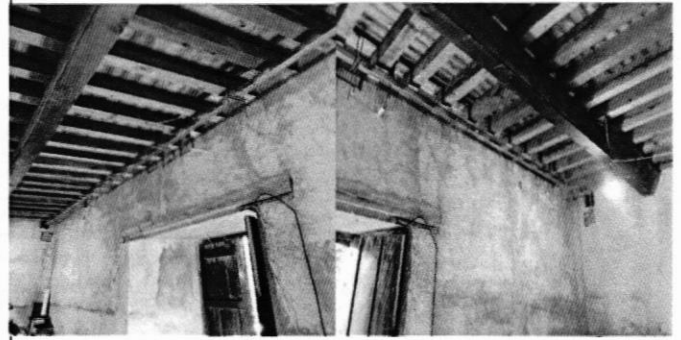
Se esta instalando canaleta para el sistema de datos
