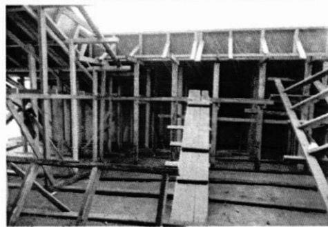
Encofrado de vigas Edificio de Aulas No. 1
