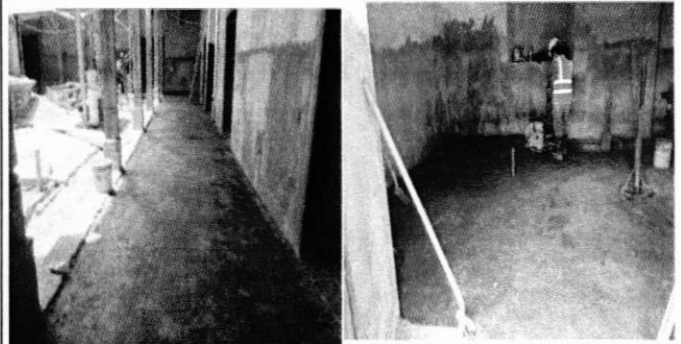
Se trabaja en la compactación de material selecto para posteriormente instalar firme de concreto para pisos.
