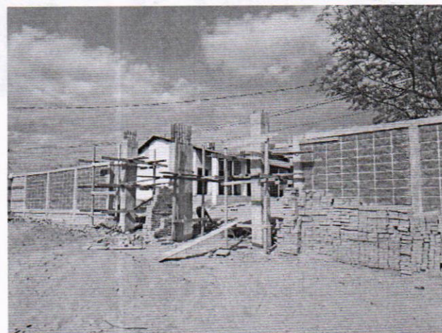
Construcción de pórtico principal
