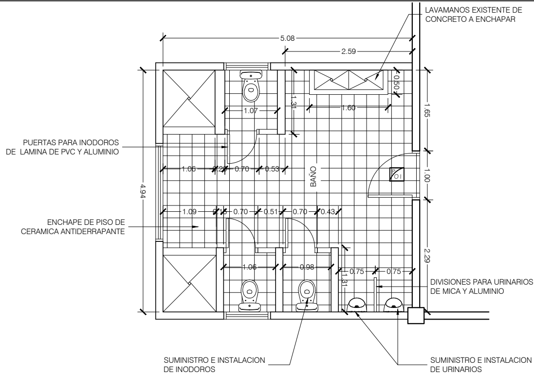
1 PLANTA DE MODULO DE BAÑOS 1:75
