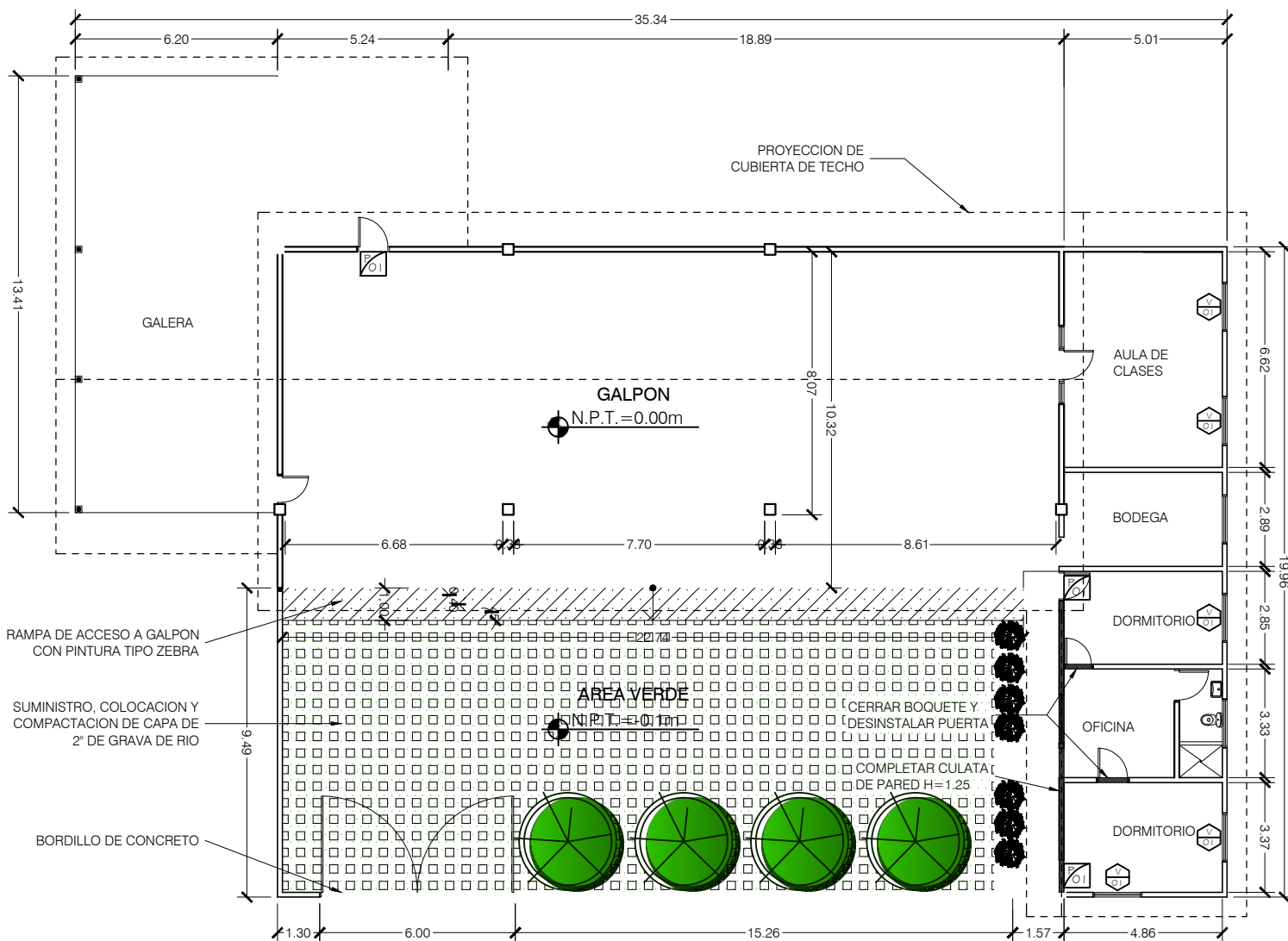
1 PLANTA DE LEVANTAMIENTO CONSTRUCTIVA
