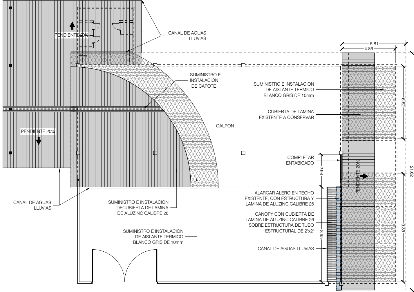
1 PLANTA CONSTRUCTIVA DE CUBIERTA DE TECHO 1:200
