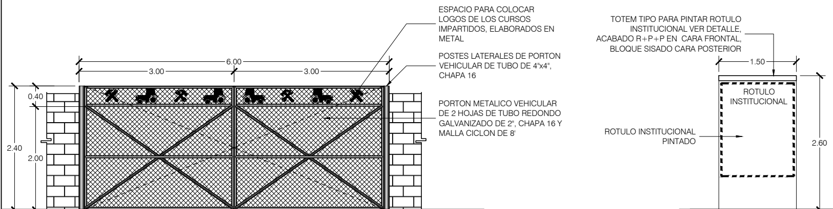
1 ELEVACION FRONTAL 1:200
