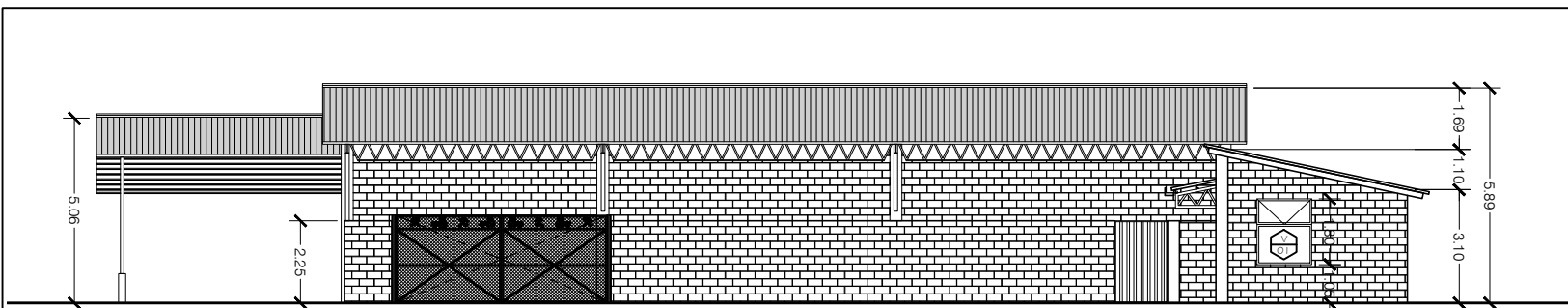
1 ELEVACION FRONTAL 1:200
