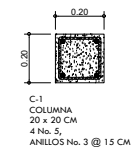
DETALLE COLUMNA C1
