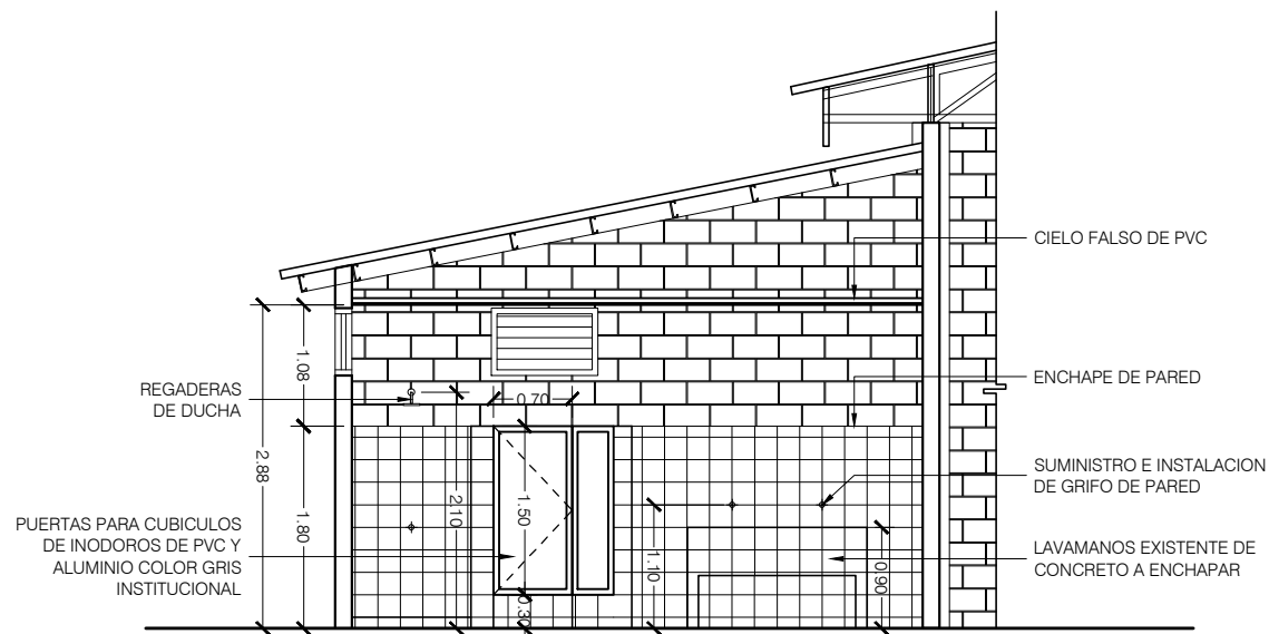
1 SECCION B-B MODULO DE BAÑOS 1:75
