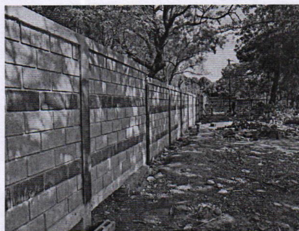
Tallado y pulido de castillos y vigas muro perimetral - Aduana Guasaule.
