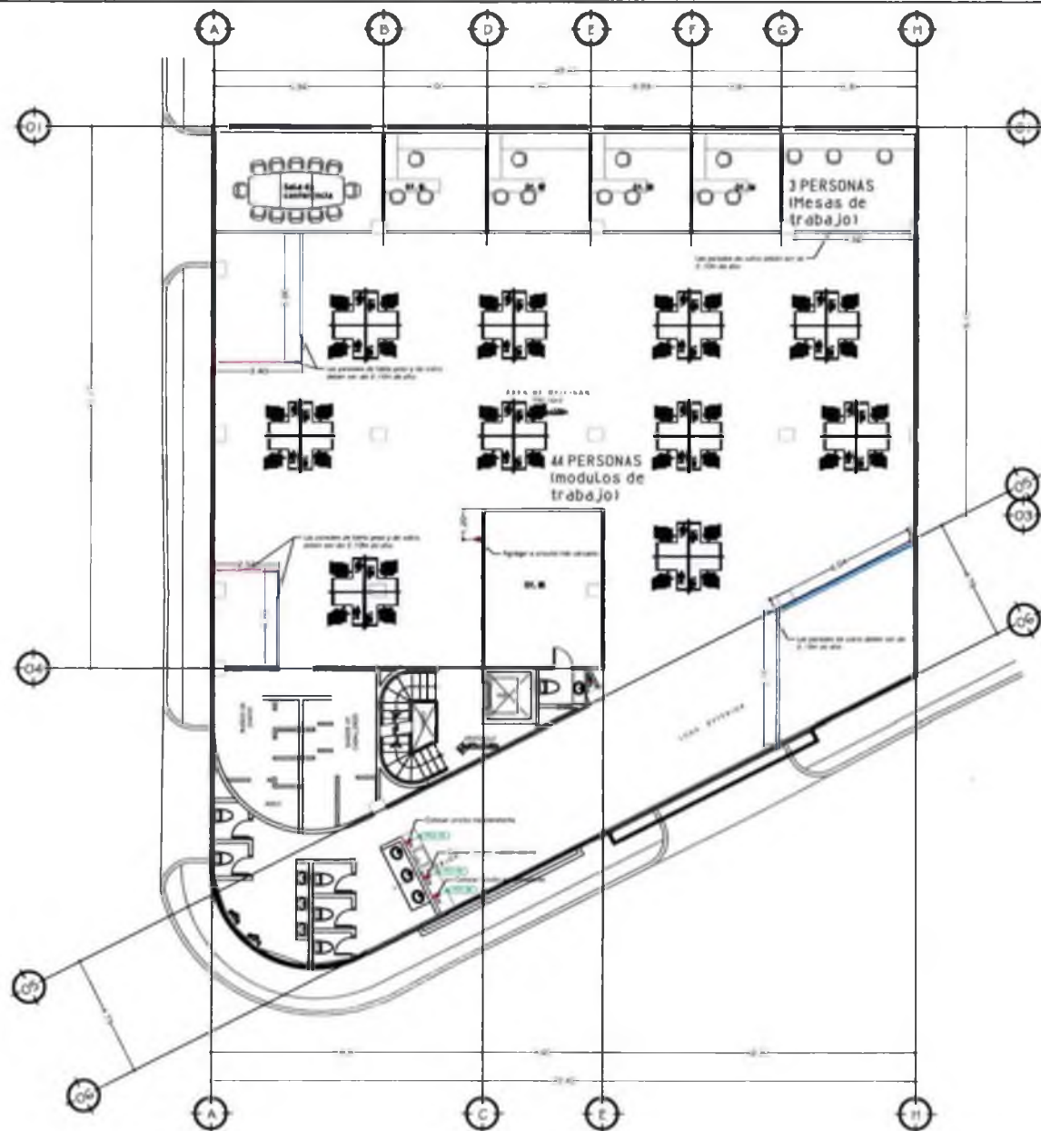
Planta arquitectónica del primer nivel
