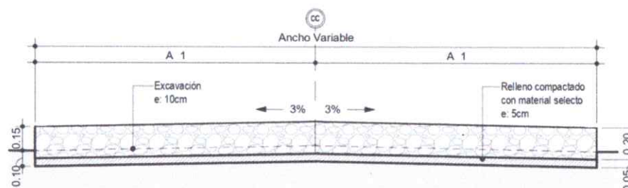
CORTE B-B PAVIMENTO DE CONCRETO CICLÓPEO
