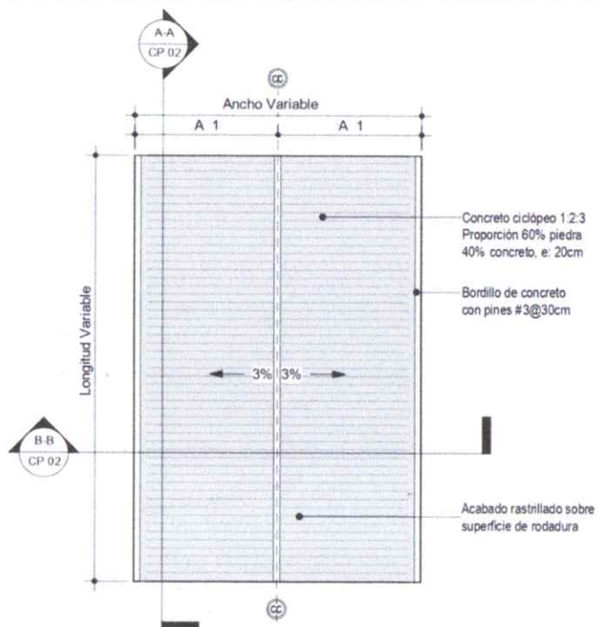
PLANTA PAVIMENTO DE CONCRETO CICLÓPEO
