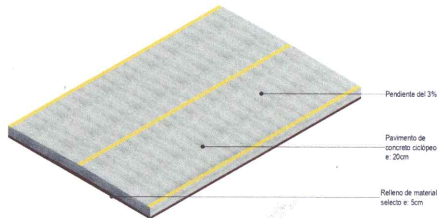
AXONOMÉTRICO PAVIMENTO DE CONCRETO CICLÓPEO
