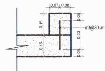
DETALLE DE BORDILLO
