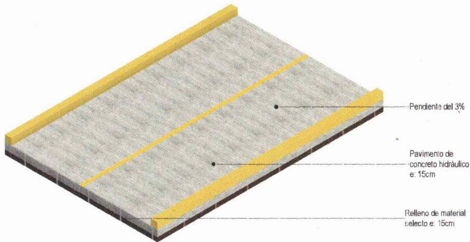
3D PAVIMENTO DE CONCRETO HIDRÁULICO
