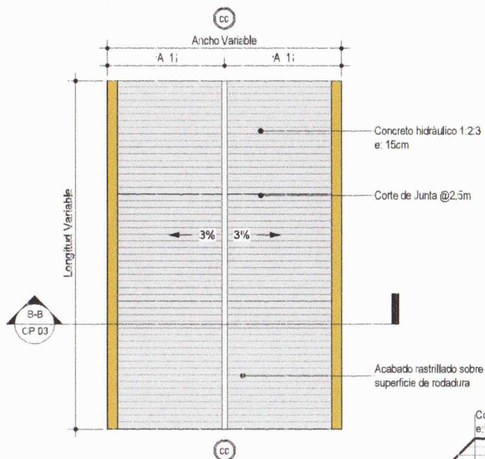
PLANTA PAVIMENTO DE CONCRETO HIDRÁULICO
