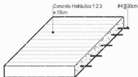
DETALLE ISOMÉTRICO DE PASAJUNTAS
