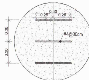
DETALLE EN PLANTA DE PASAJUNTAS
