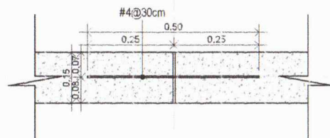
DETALLE TRANSVERSAL DE PASAJUNTAS
