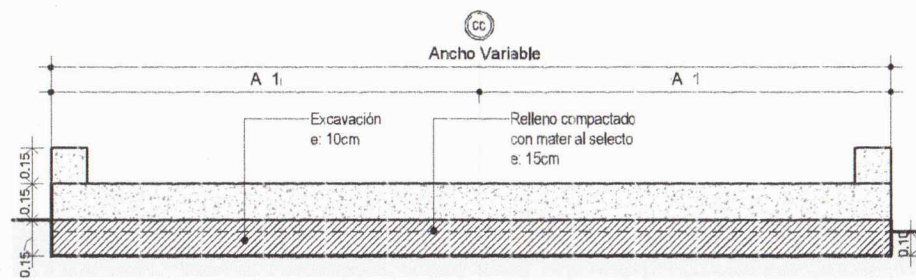
CORTE B-B PAVIMENTO DE CONCRETO HIDRÁULICO
