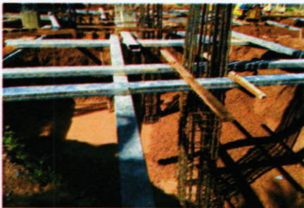
Zapatas (3) de Concreto y armado de pedestales (Grupo Sur-Este). (31-1-2017)
