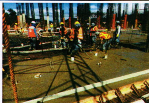
Fundición de sección de losa de Nivel 1.
