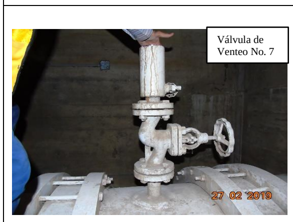
Válvula de Venteo No. 7 en el Segmento 2211
