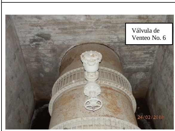
Válvula de Venteo No. 6 en el Segmento 2012
