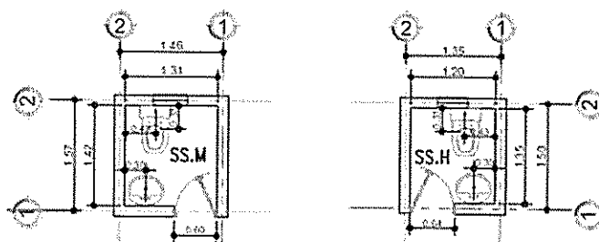
PLANO DE UBICACIÓN DE MOBILIARIO SANITARIO
