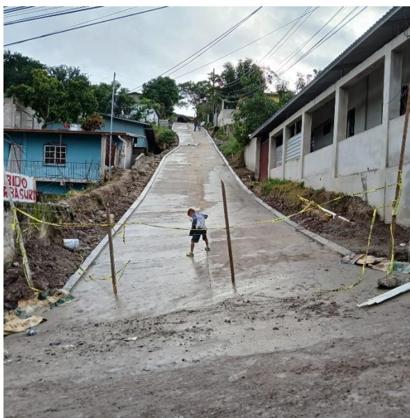
Proyecto finalizado de pavimentación de calle barrio Bella Vista, pendiente Doña Ticha, La Entrada, Nueva Arcadia, Copán.
