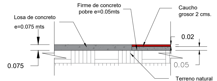
DETALLE DE CAUCHO EN ÁREA DE JUEGOS
