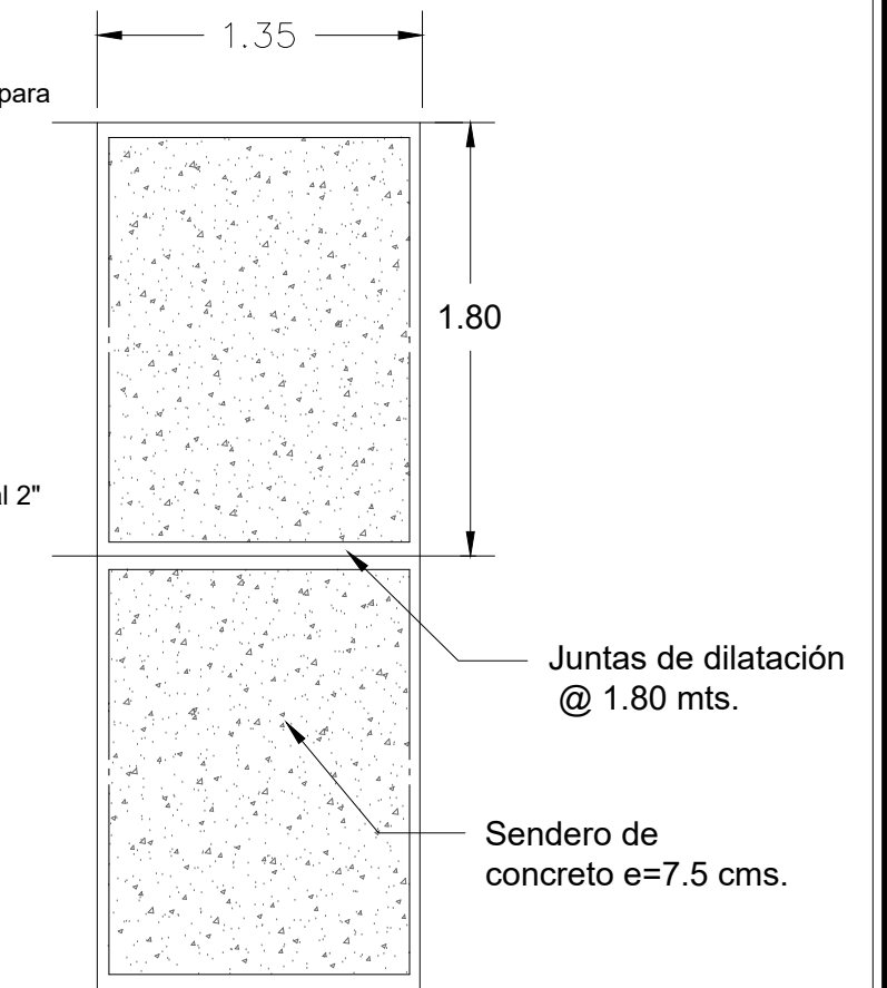
PLANTA DE SENDERO ESC. 1:35
