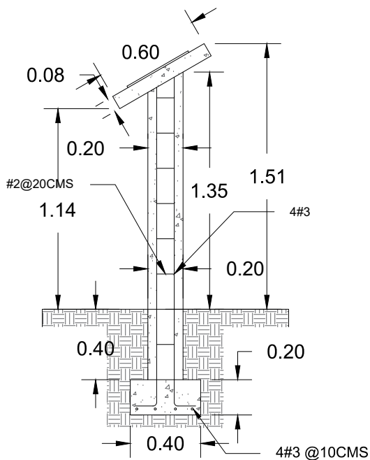
DETALLE DE PLACA DE MÁRMOL ESC.1:30
