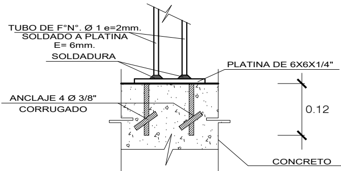
DETALLE DE ANCLAJE DE BARANDA
