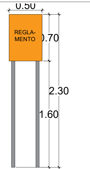
RÓTULO DE AVISO ESC. 1:30
