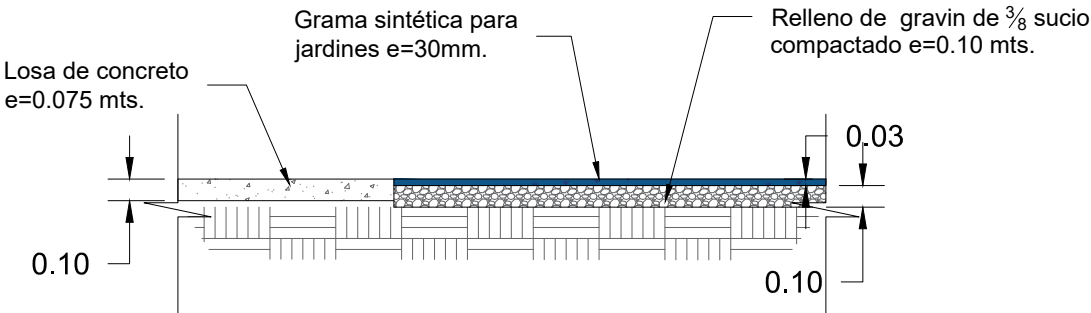
DETALLE DE GRAMA SINTÉTICA
