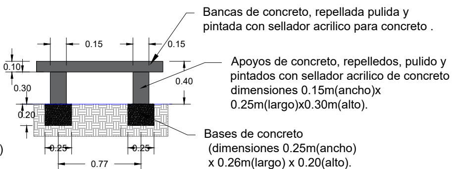
DETALLE DE BANCAS DE CONCRETO (quisco)
