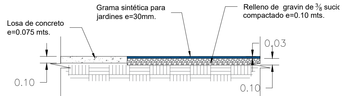
DETALLE DE GRAMA SINTÉTICA
