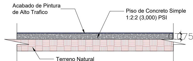
DETALLE DE FIRME DE CONCRETO
