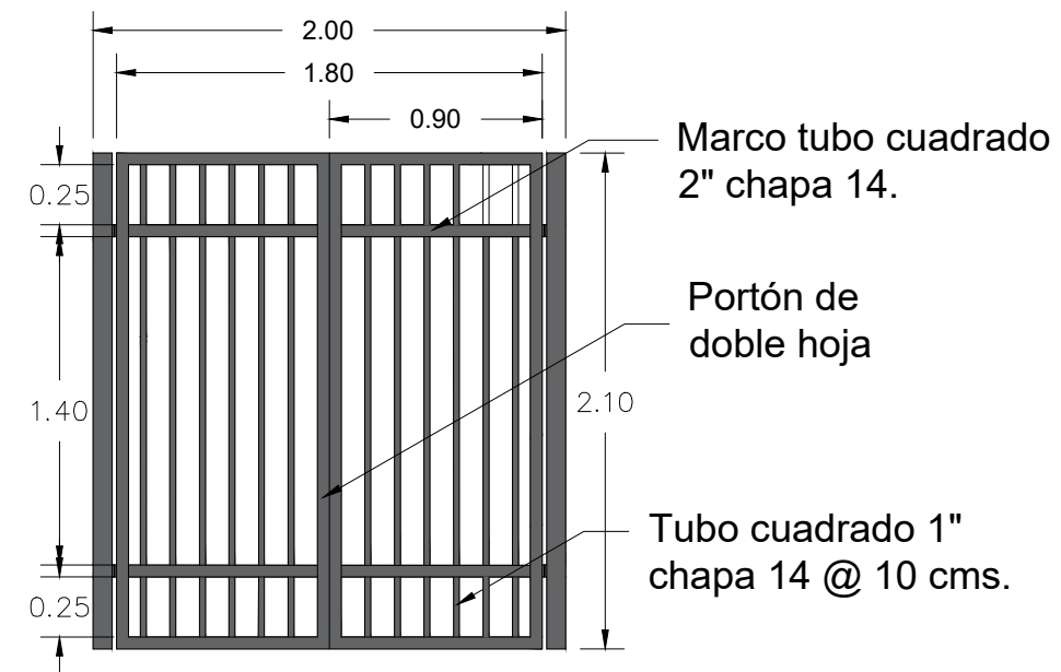
DETALLE DE PORTON ESC. 1:35
