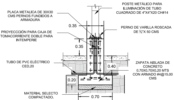
DETALLE DE CIMENTACIÓN POSTE ELECTRICO ESC. 1:50
