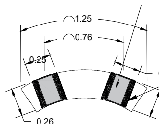
DETALLE DE BANCAS DE CONCRETO (quisco)
