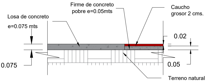
DETALLE DE CAUCHO EN ÁREA DE JUEGOS
