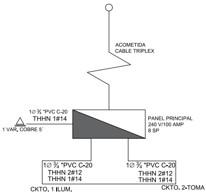
DIAGRAMA UNIFILAR ESC. 1:35
