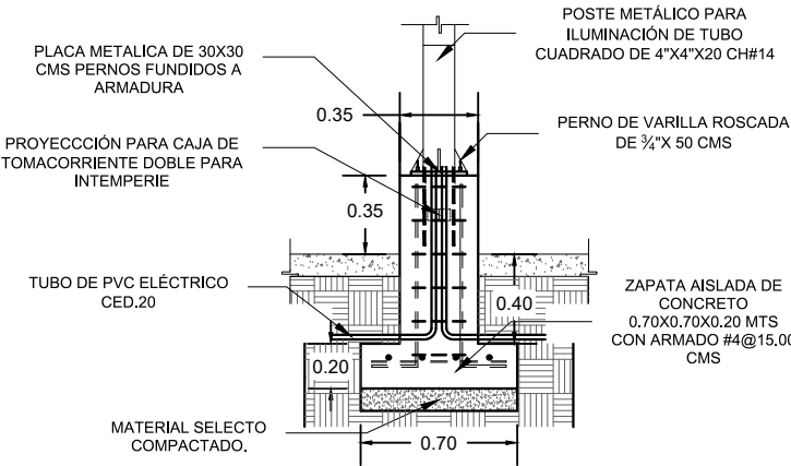
DETALLE DE CIMENTACIÓN POSTE ELECTRICO ESC. 1:50
