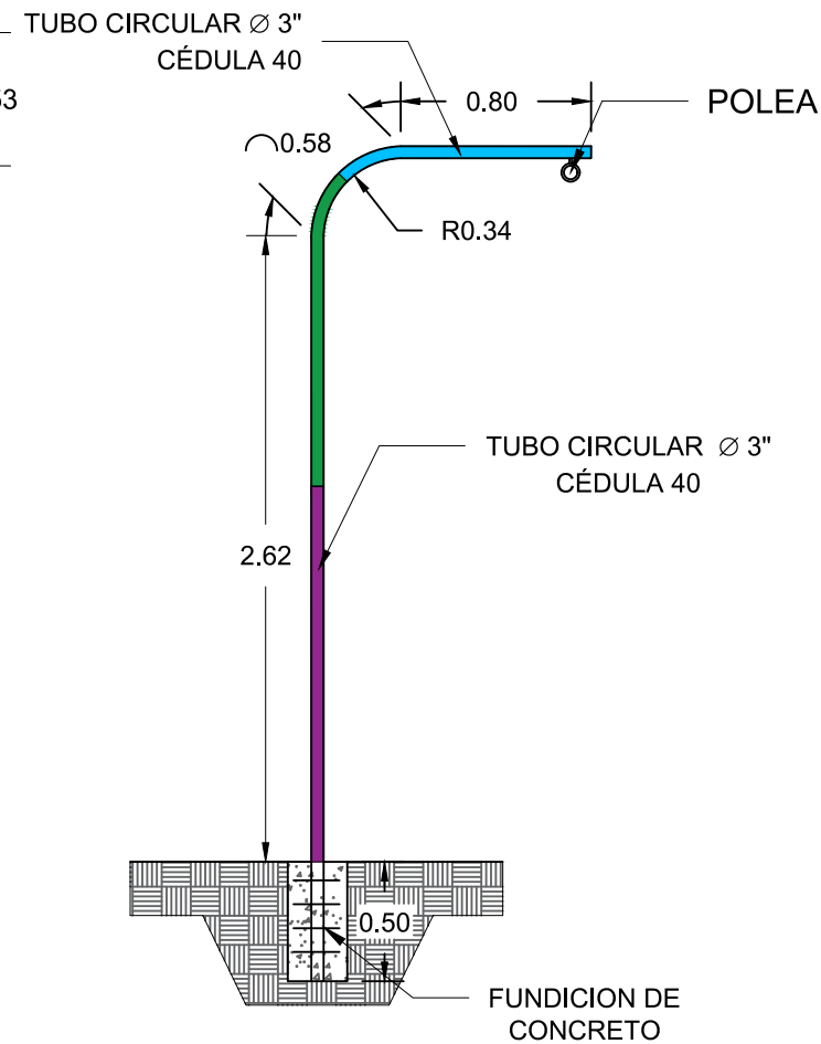
POSTE PARA PIÑATAS ESC. 1:35
