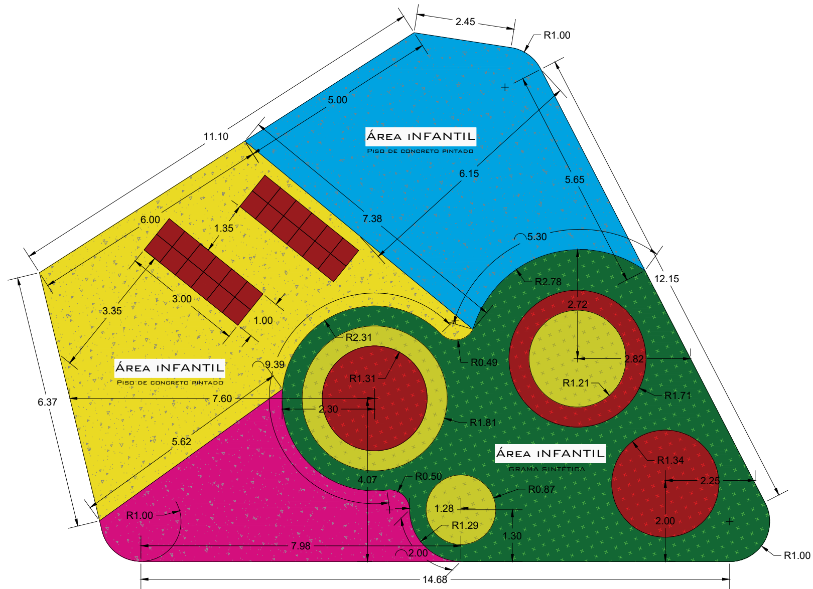
PLANTA JUEGOS INFANTILES
