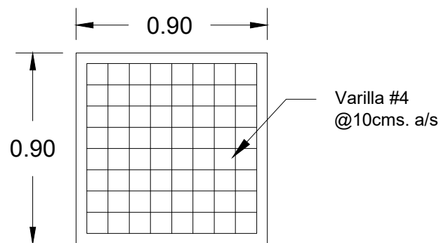
ZAPATA AISLADA ESC.1:35
