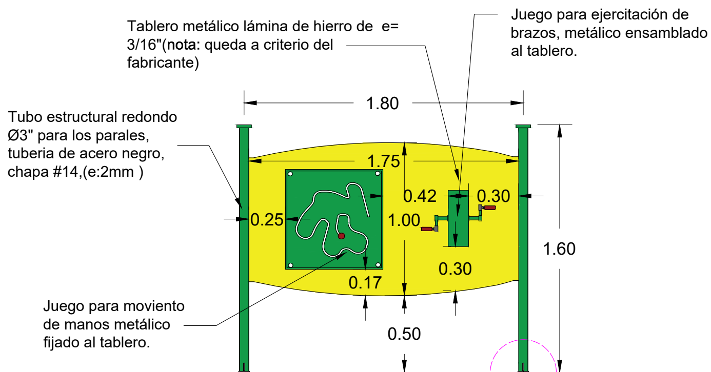
DETALLE D-01 TABLERO FISICO-MOTOR ESC. 1:25
