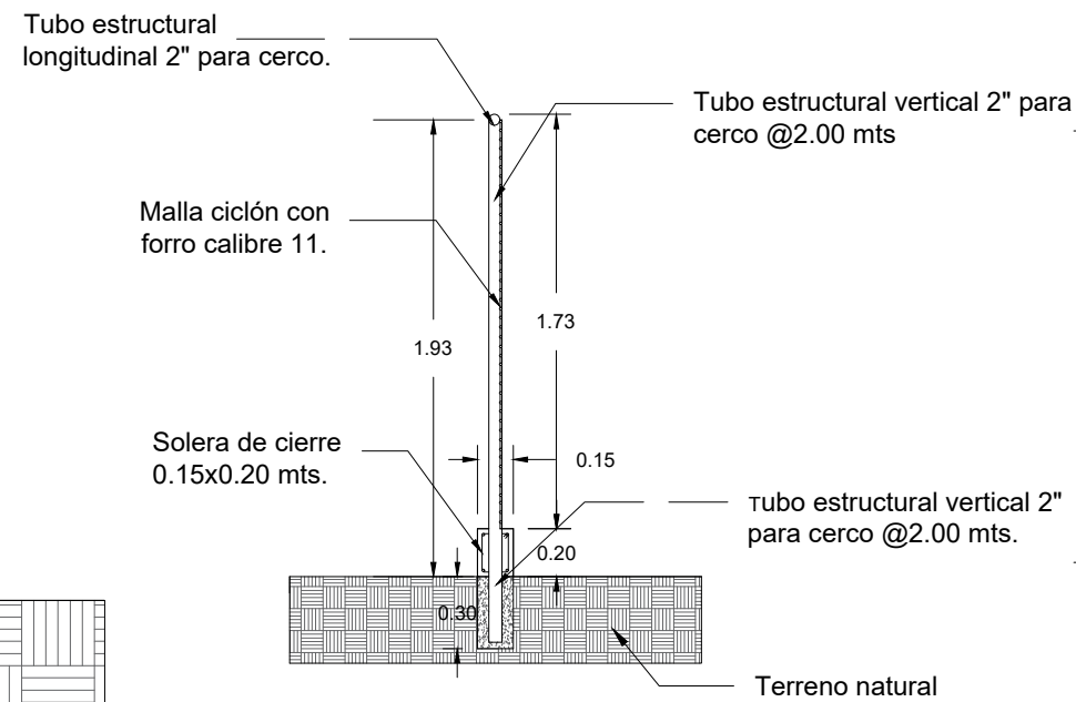
DETALLE A-A ESC.1:50
