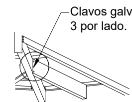
FIJADO TECHO DE MADERA
