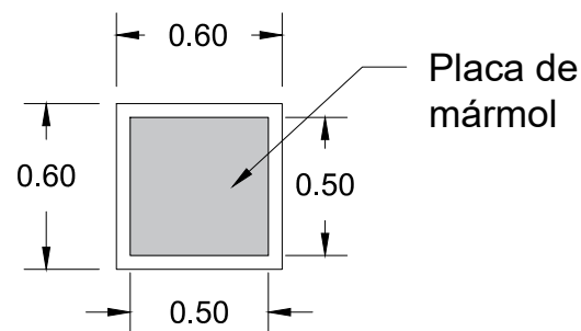
PLANTA DE PLACA DE MÁRMOL ESC.1:30
