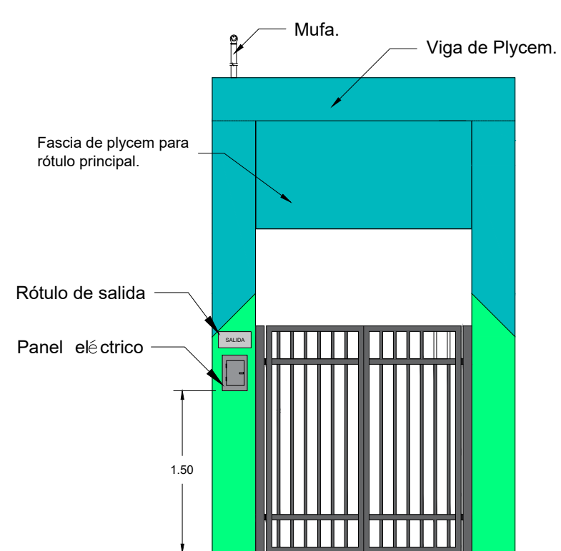
DETALLE DE ACCESO POSTERIOR ESC.1:50
