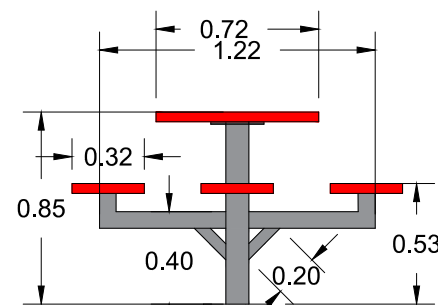
ELEVACIÓN MESAS DE AJEDREZ ESC. 1:35
