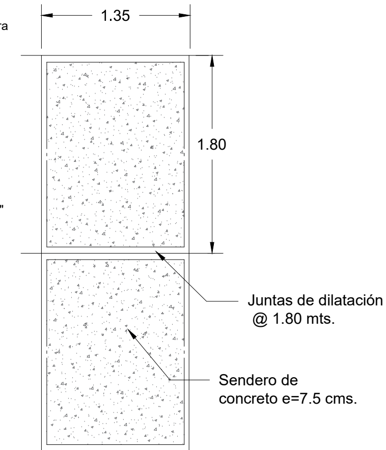
PLANTA DE SENDERO ESC. 1:35
