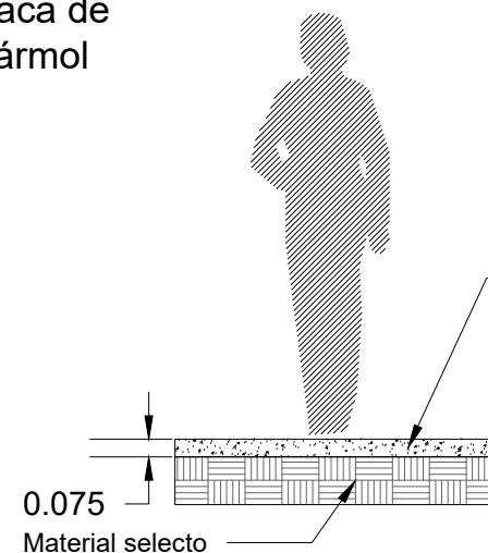
ELEVACIÓN DE SENDERO ESC. 1:35
