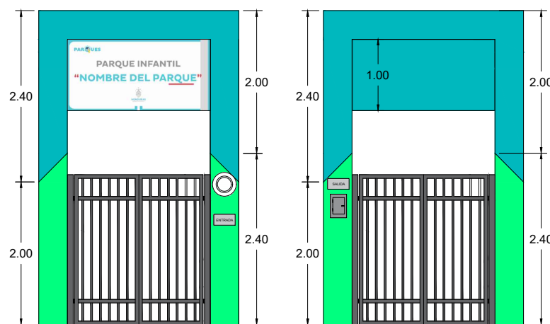
DETALLE DE ACCESO FRONTAL (pintura) ESC.1:75
