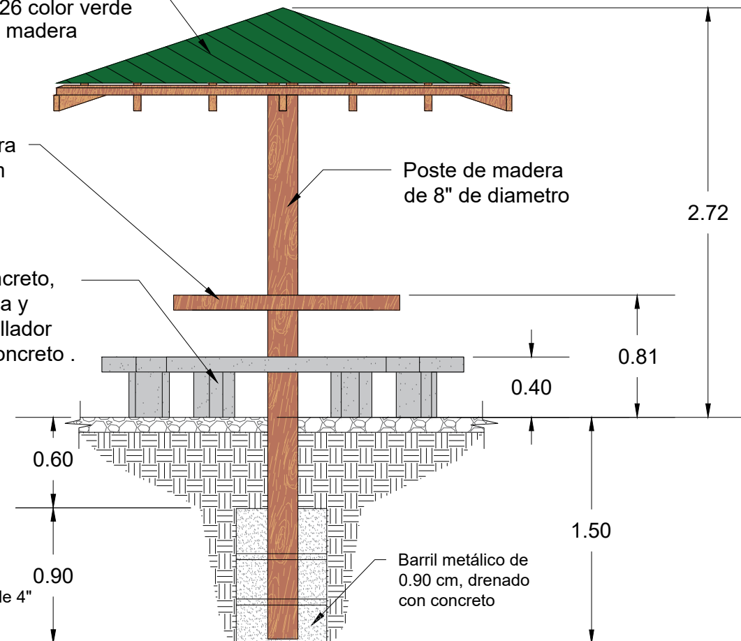
DETALLE DE QUIOSCO
