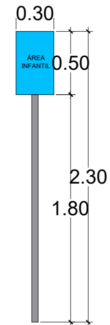
ROTULO DE SEÑALAMIENTO DE ÁREA ESC. 1:30
