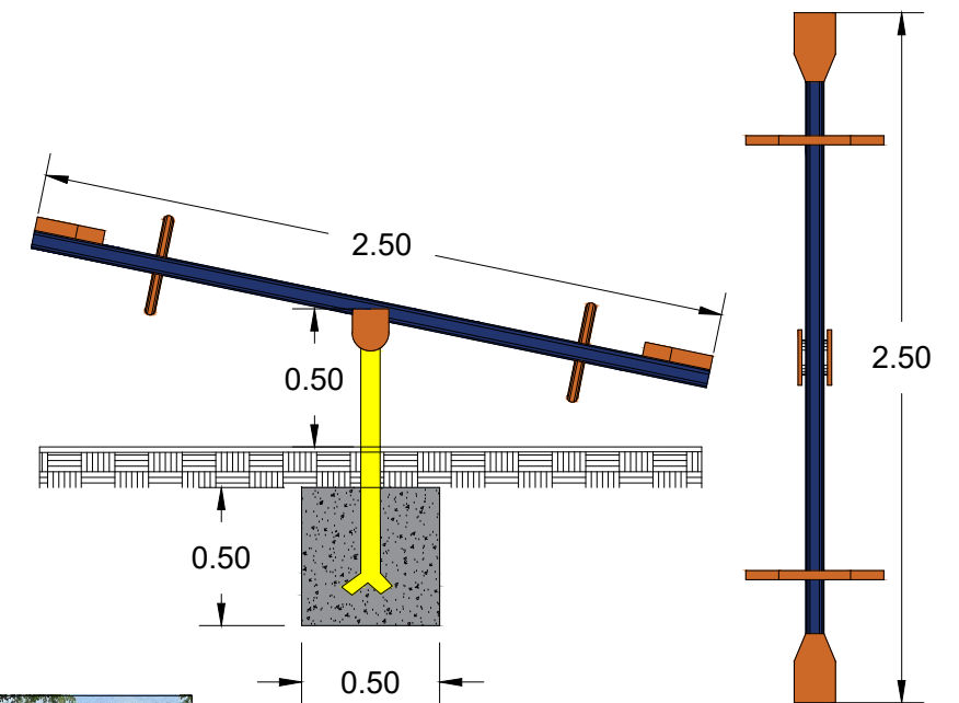
SUBE Y BAJA ESC. 1:35
