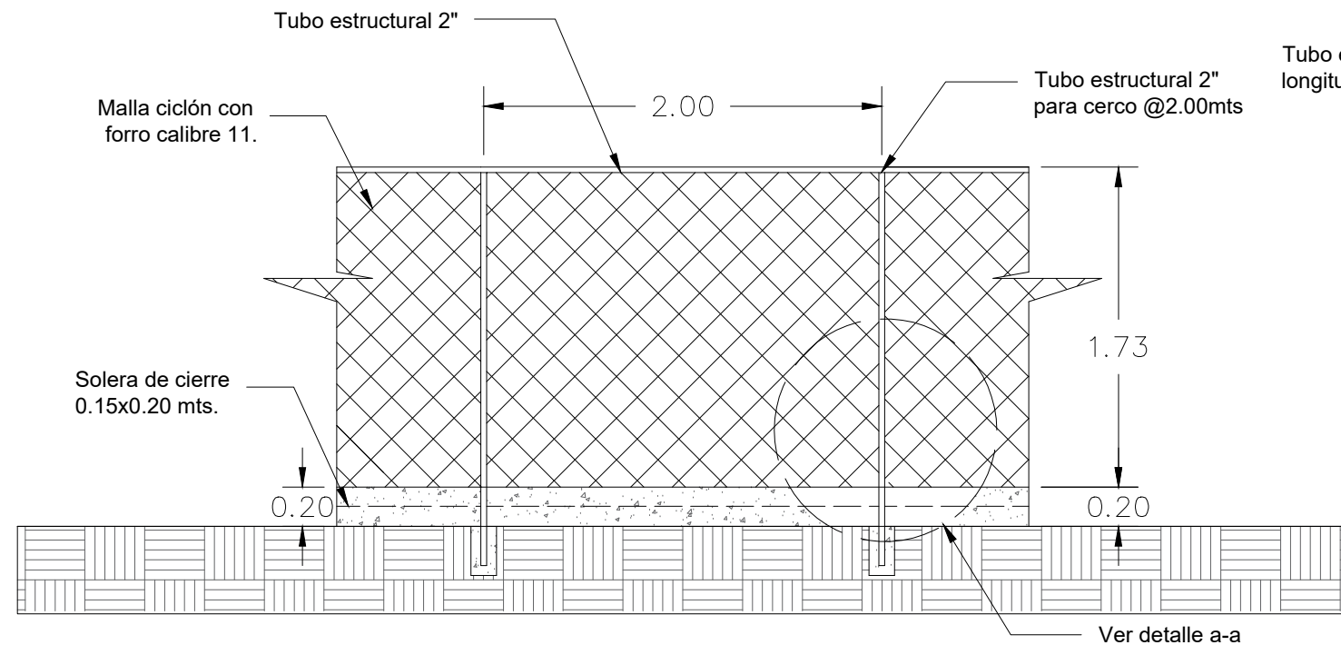
ELEVACIÓN DE CERCO ESC.1:35
