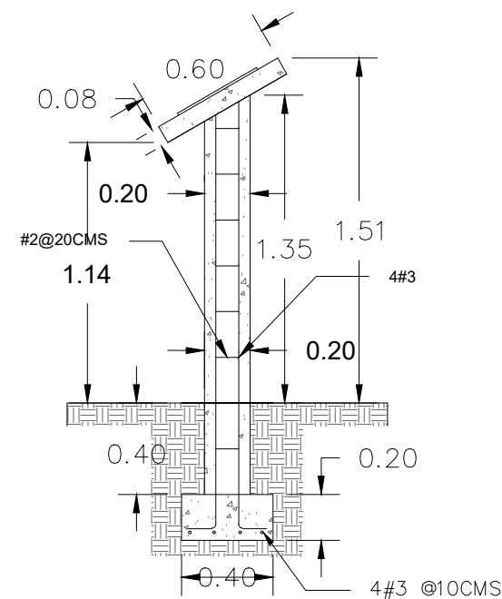
DETALLE DE PLACA DE MÁRMOL ESC.1:30
