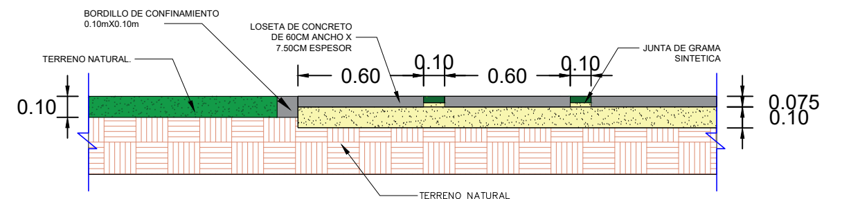
DETALLE DE BORDILLO DE CONFINAMIENTO Área social ESC. 1:25
