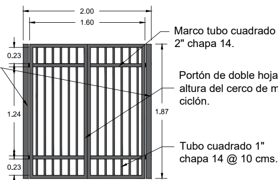
DETALLE DE PORTÓN SECUNDARIO ESC. 1:35
