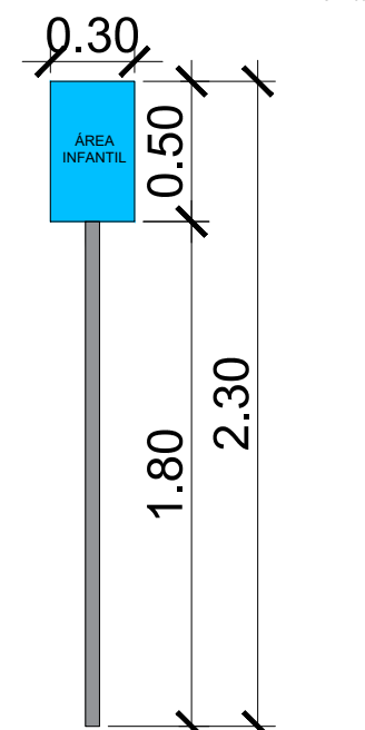
ROTULO DE SEÑALAMIENTO DE ÁREA ESC. 1:30
