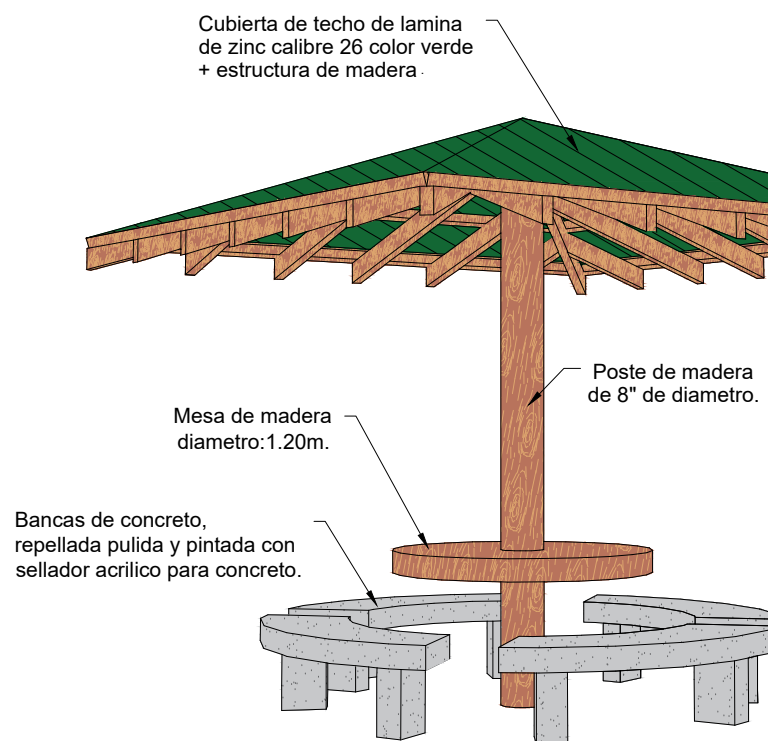
DETALLE DE QUIOSCO
