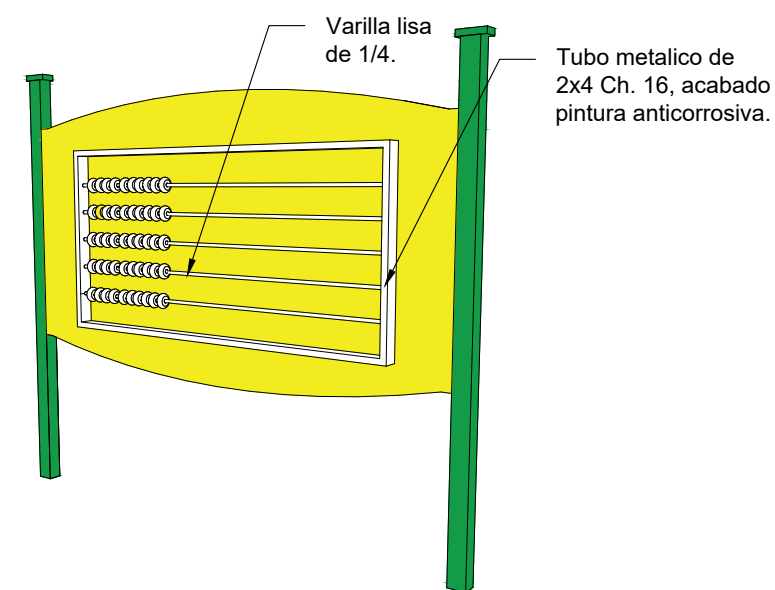
DETALLE DE TABLERO FISICO MOTOR ESC. 1:25
