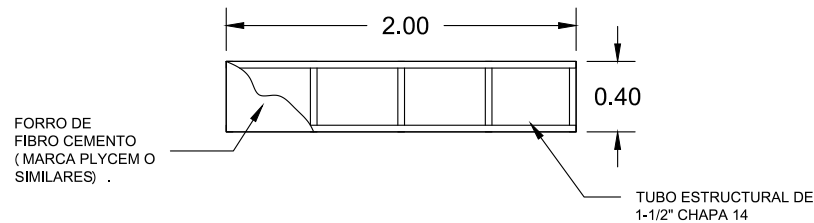
DETALLE FASCIA DE ACCESO ESC. 1:50
