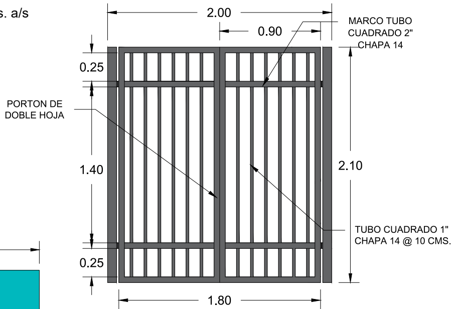
DETALLE DE PORTON ESC. 1:35
