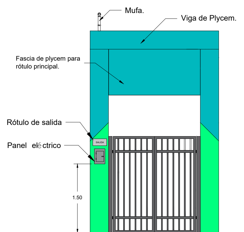
DETALLE DE ACCESO POSTERIOR
