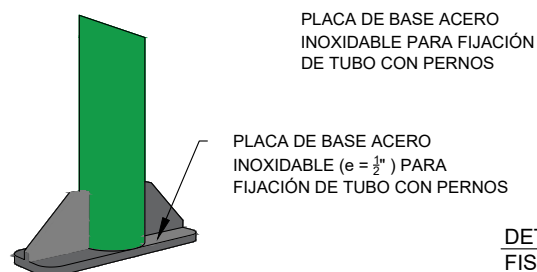
DETALLE D-01 TABLERO FISICO-MOTOR ESC. 1:25
