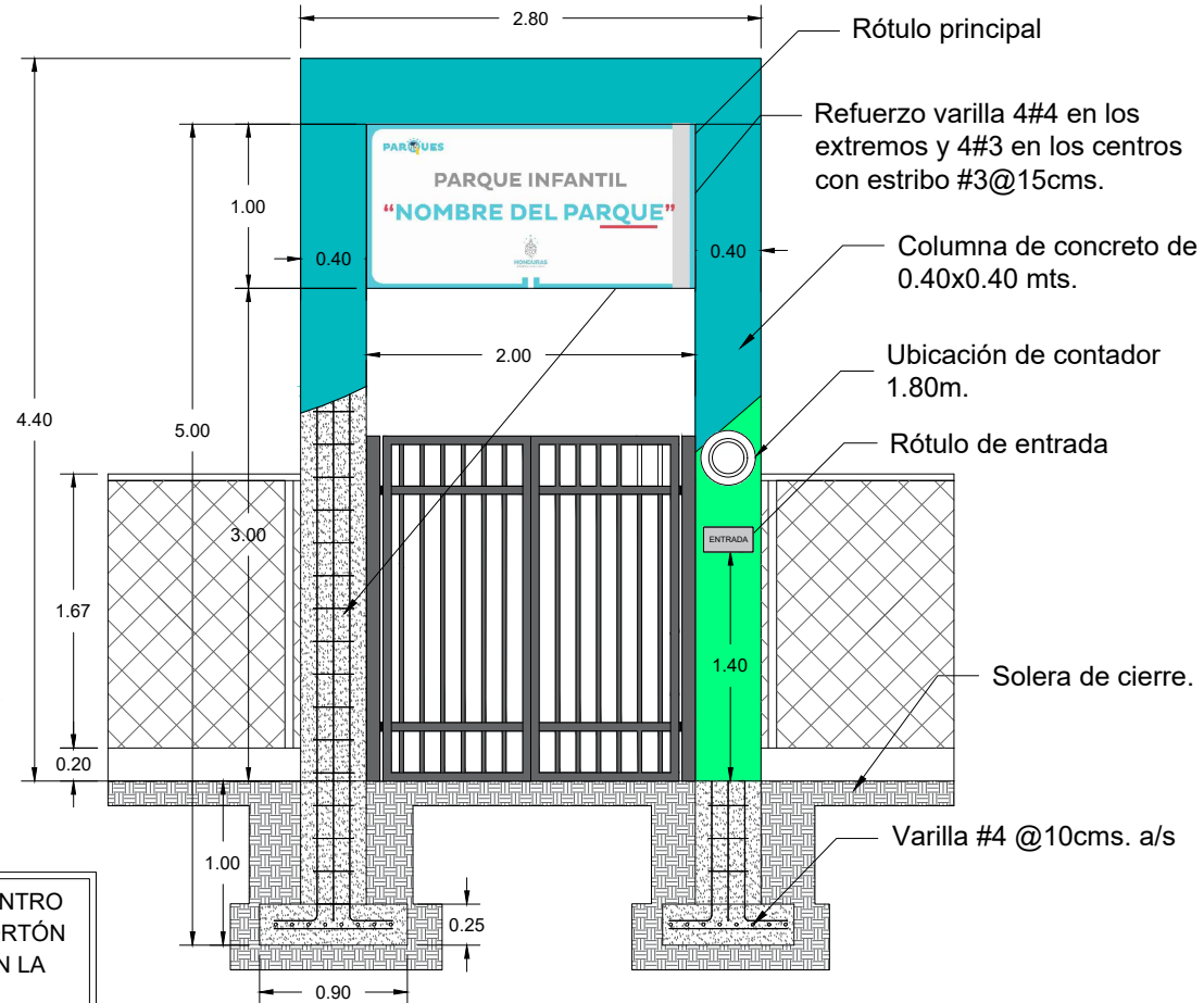
DETALLE DE ACCESO FRONTAL
