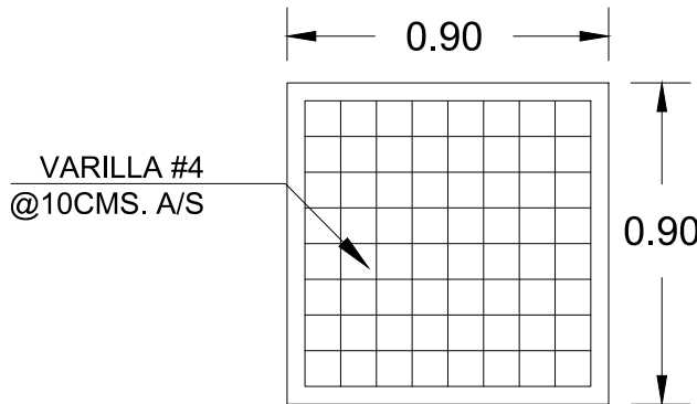
ZAPATA AISLADA ESC.1:20
