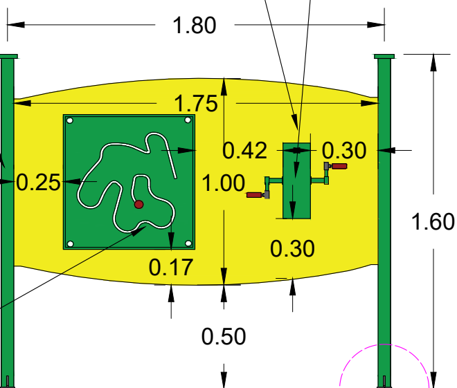
DETALLE DE TABLERO FISICO MOTOR ESC. 1:25
