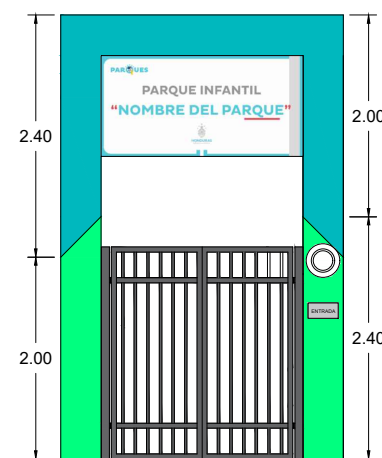
DETALLE DE ACCESO FRONTAL (pintura)
