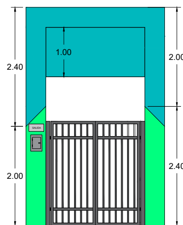
DETALLE DE ACCESO POSTERIOR (pintura)
