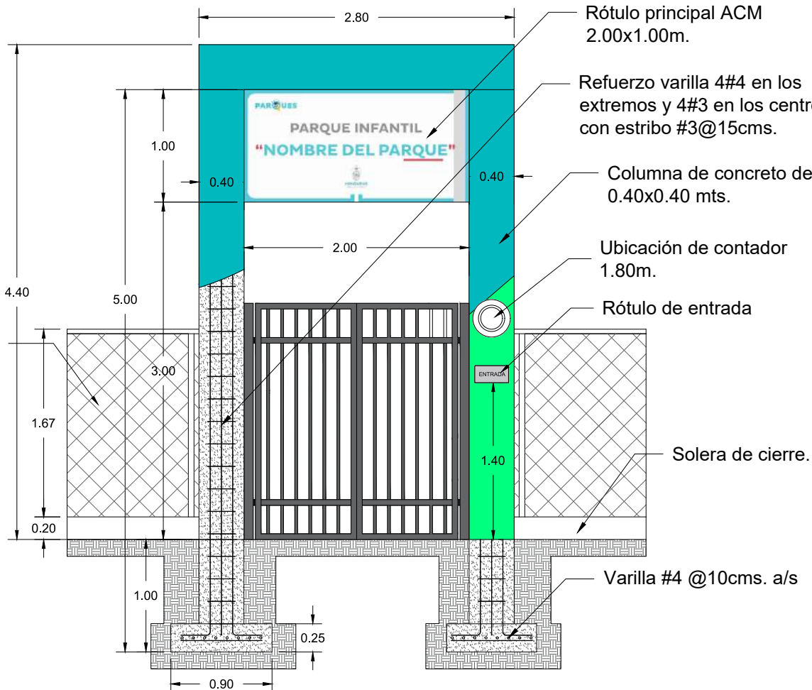
DETALLE DE ACCESO FRONTAL ESC.1:50
