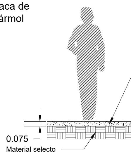
ELEVACIÓN DE SENDERO ESC. 1:35
