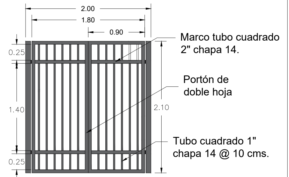
DETALLE DE PORTON
