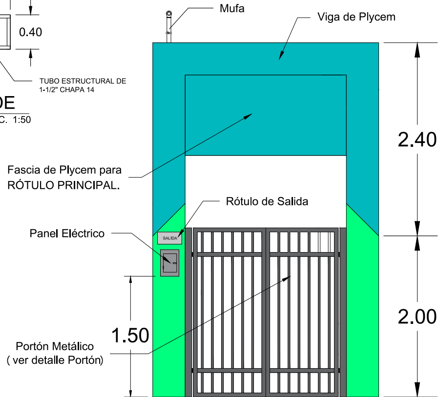
DETALLE DE ACCESO POSTERIOR ESC.1:50
