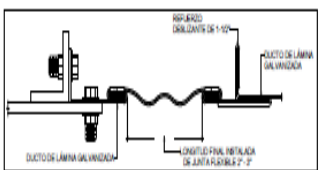
D INSTALACIÓN DE CONECTOR FLEXIBLE EN EQUIPO
