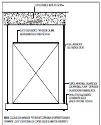
H SOPORTE DE DUCTO RECTANGULAR BAJO LOSA
