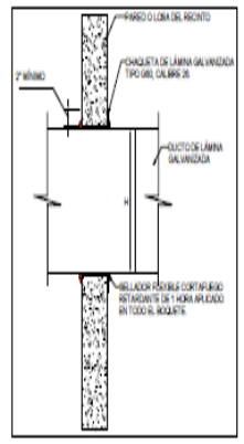
F PASANTE DE DUCTOS A TRAVÉS DE PAREDES
