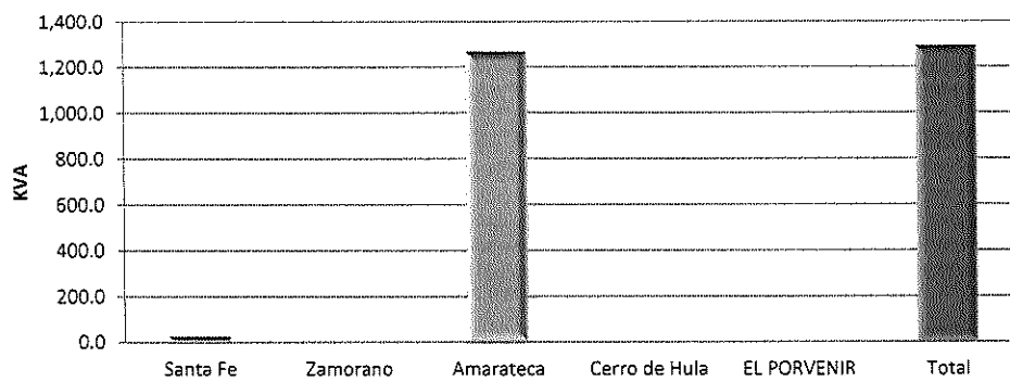
CAPACIDAD INSTALADA EN 34.5 KV
