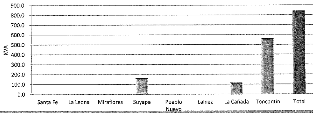
CAPACIDAD INSTALADA EN 13.8 KV
