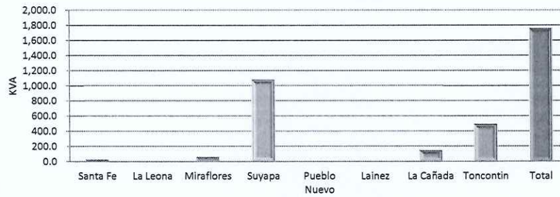
DEMANDA PROYECTADA POR DISEÑOS EN 13.8 KV
