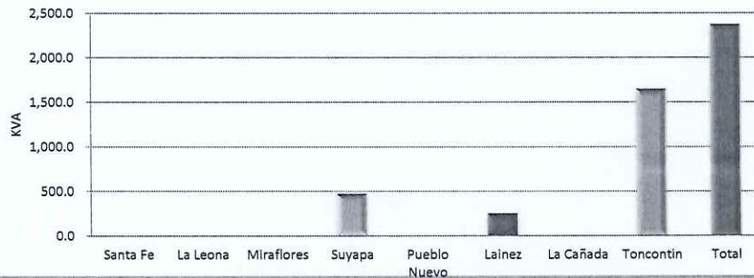
CAPACIDAD INSTALADA EN 13.8 KV
