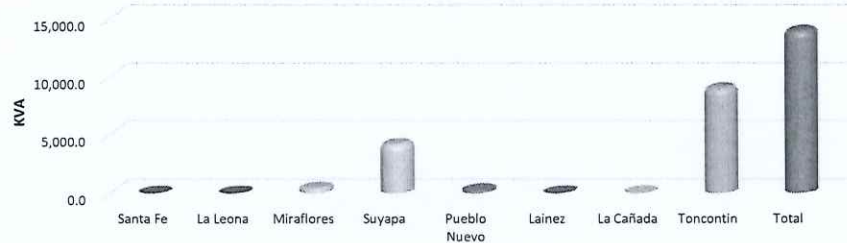
DEMANDA PROYECTADA POR FACTIBILIDAD EN 13.8 KV
