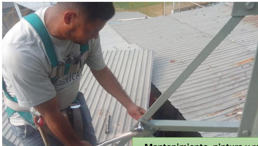
Mantenimiento, pintura y reforzamiento de Torres de Iluminación de Estadio Excelsior.
