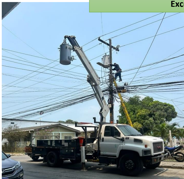
Reparación de Sistema Eléctrico e instalación de Transformador para Locales de Estadio Excélsior.
