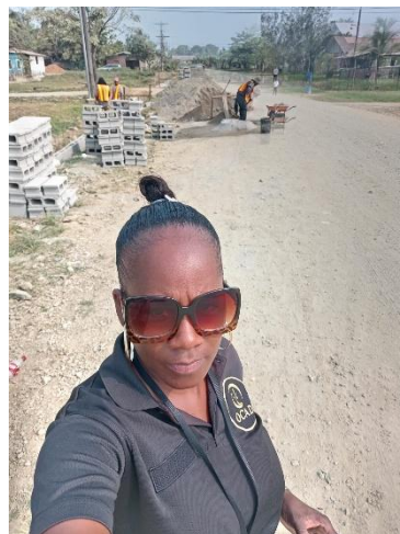
Construcción de Cunetas Pluviales 8.00 a.m. Las Palmas, 24 mayo 2024 asistente Wendy Arauz
