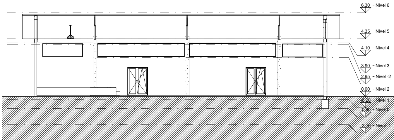
2 Sección 2 A107 1: 100
