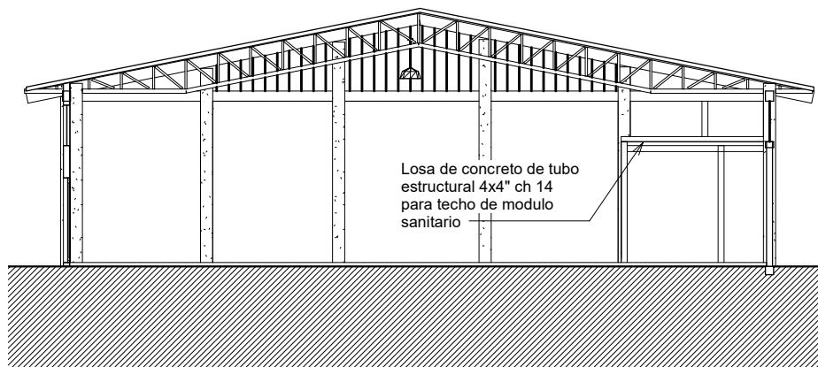
2 Sección 9 A104 1 : 100
