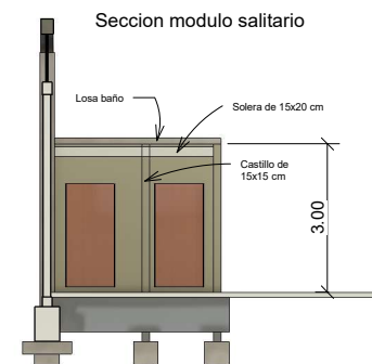
3 Sección 5 A104 1 : 100
