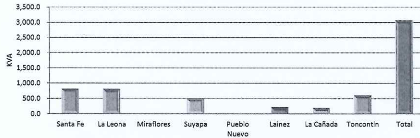
DEMANDA PROYECTADA POR DISEÑOS EN 13.8 KV
