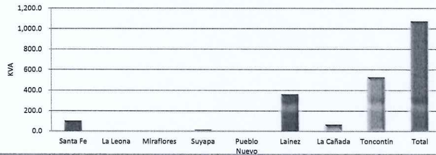
CAPACIDAD INSTALADA EN 13.8 KV
