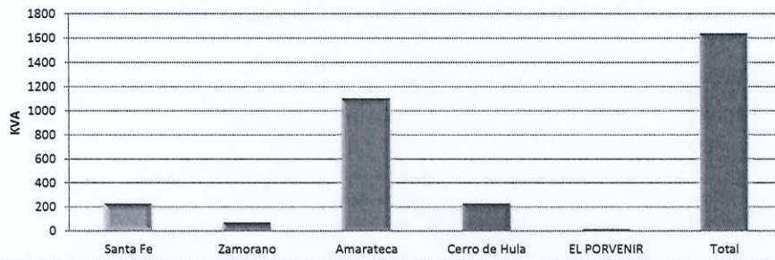
DEMANDA PROYECTADA POR DISEÑOS EN 34.5 KV
