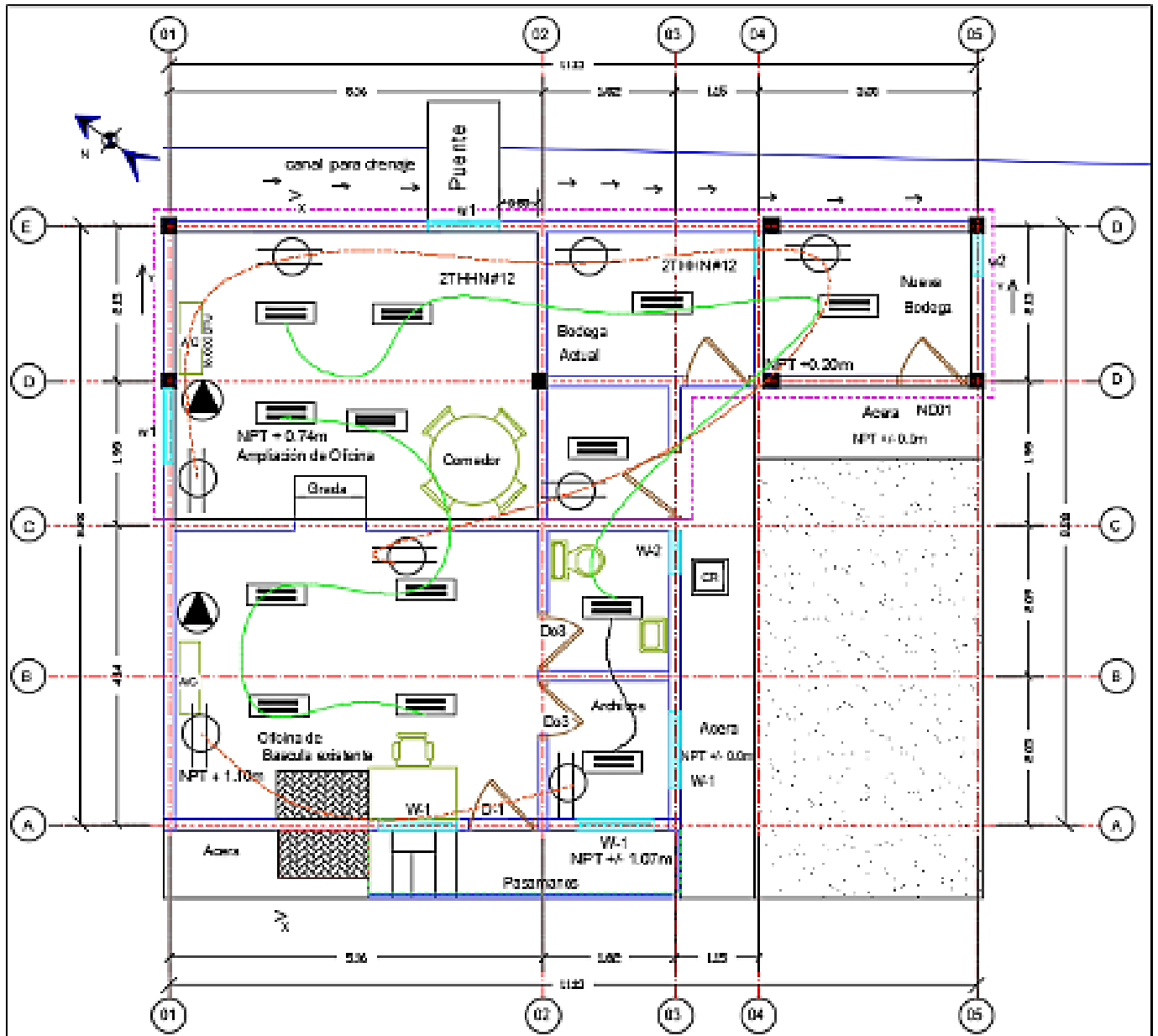
PLANO DE INSTALACIONES ELECTRICAS DEL INMUEBLE
