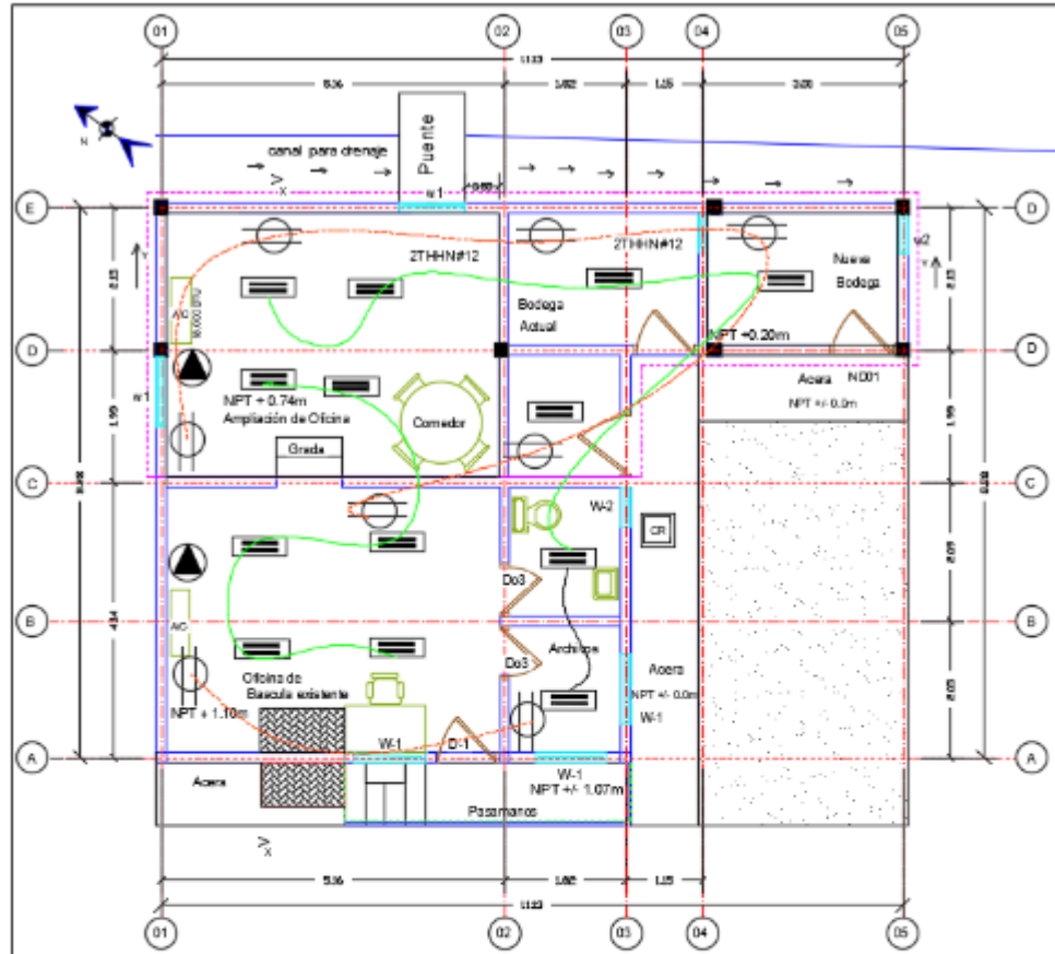
PLANO DE INSTALACIONES ELECTRICAS DEL INMUEBLE
