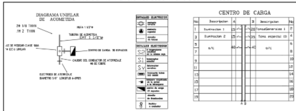
PLANO DE INSTALACIONES ELECTRICAS DEL INMUEBLE
