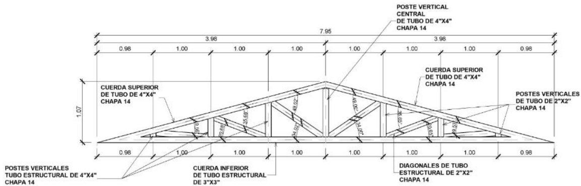
DETALLE TIJERA T-1
