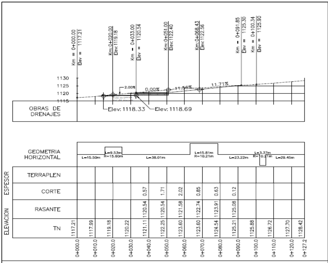
Sección del perfil longitudinal proyectado de la nueva calle donde se indica el desplante del foso de la Báscula indicándose las pendientes máximas de ascenso.
