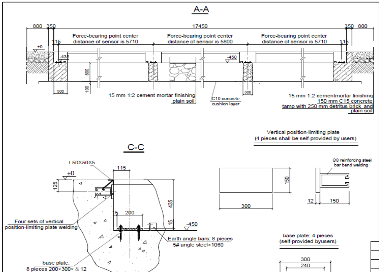
Secciones transversales de la cimentación
