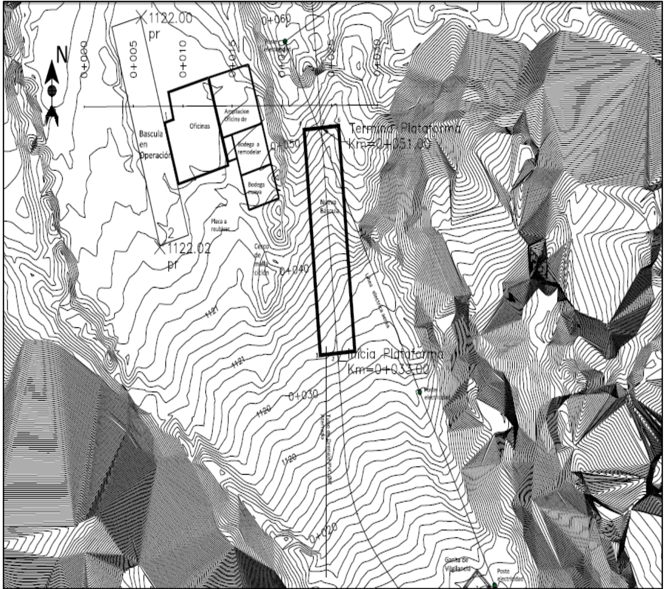
Diseño geométrico de calle de acceso, donde se reflejan las curvas de nivel del terreno caracterizando el relieve de los predios donde se emplazará la nueva bascula construir
