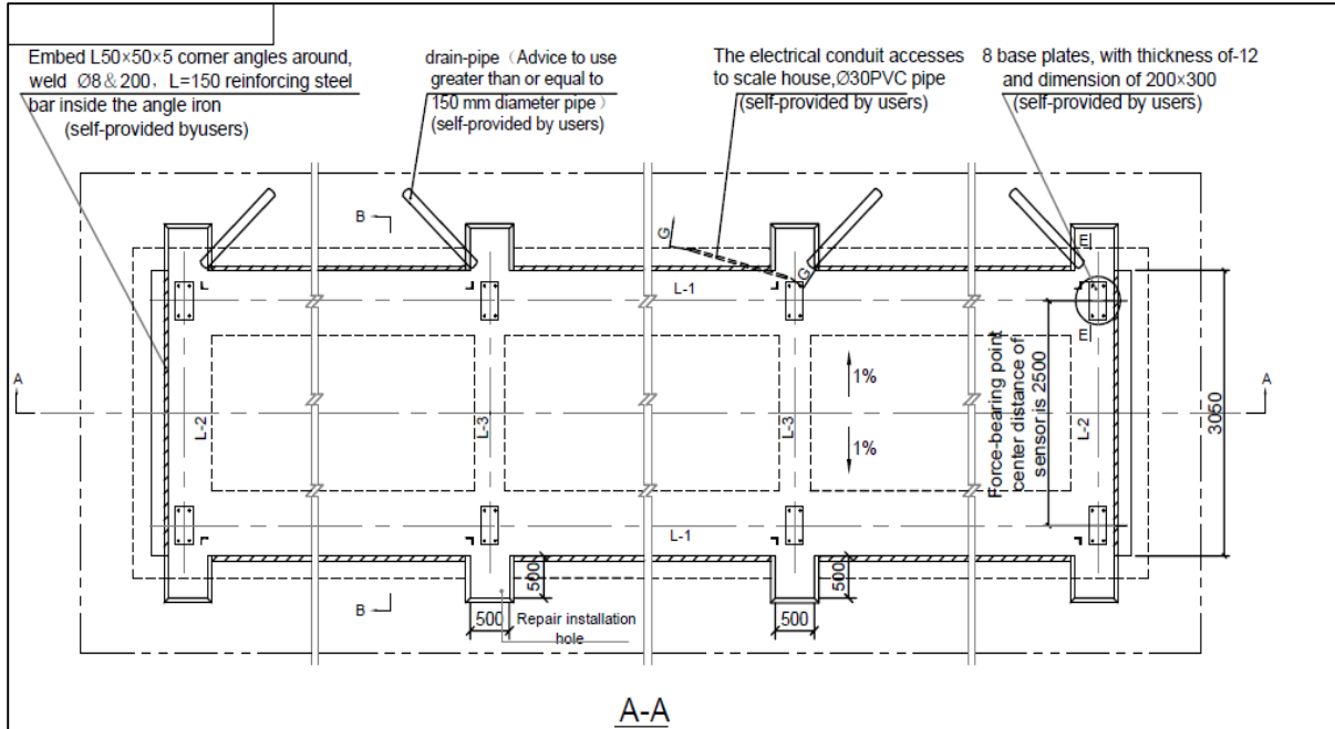
Planta de cimentación de soporte de la báscula según el proveedor
