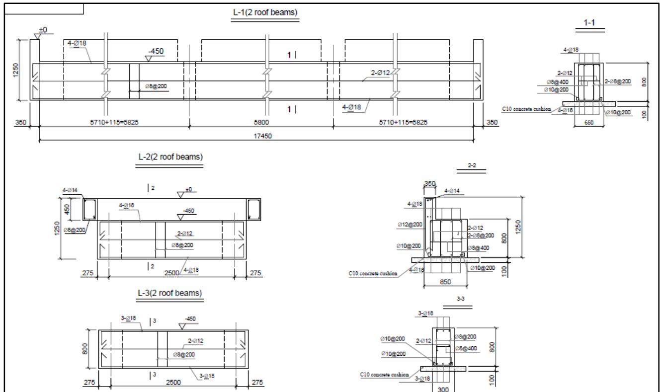
Secciones transversales de las paredes de contención de apoyo de los soportes de la báscula
