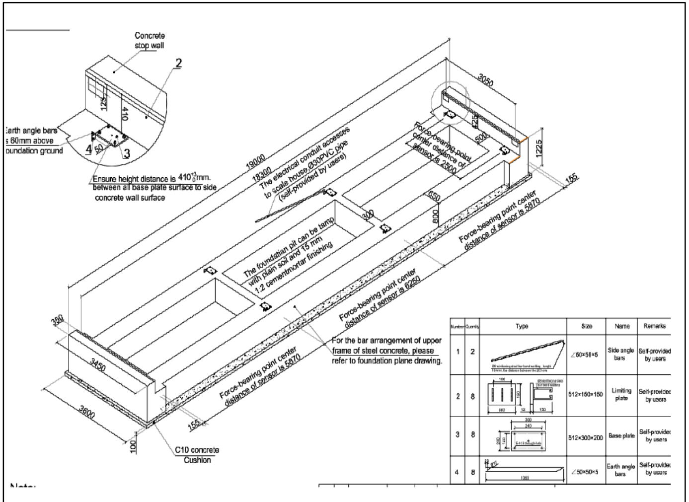
Planos de cimentación proporcionados por el proveedor de la báscula
