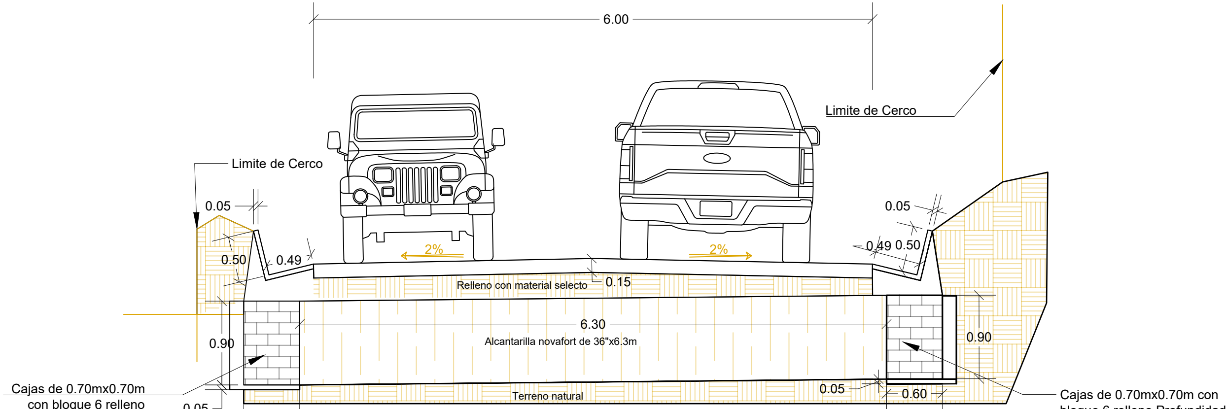
Corte Perfil de Carretera P7-P34 Escala 1:40
