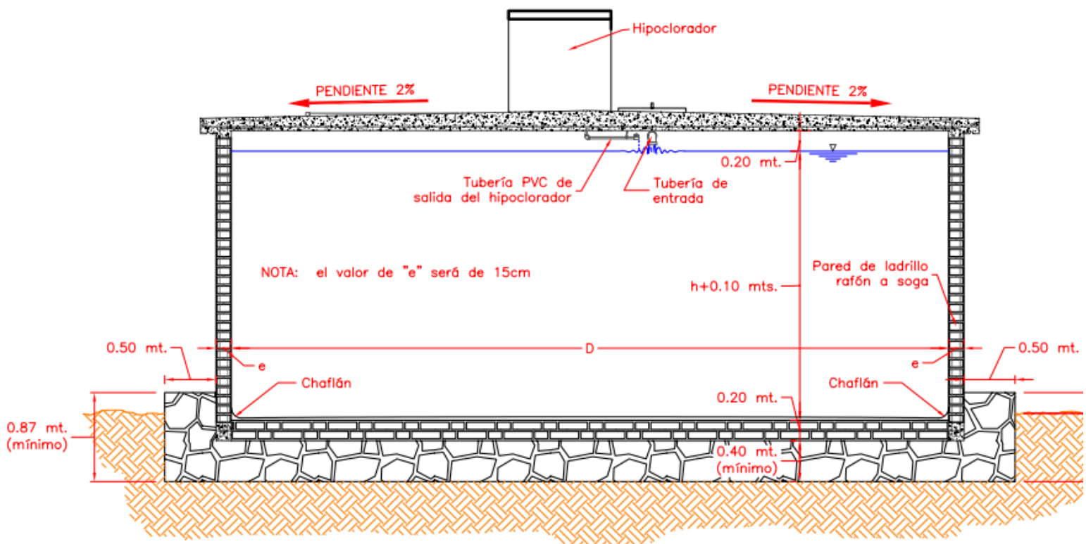
Seccion transversal
