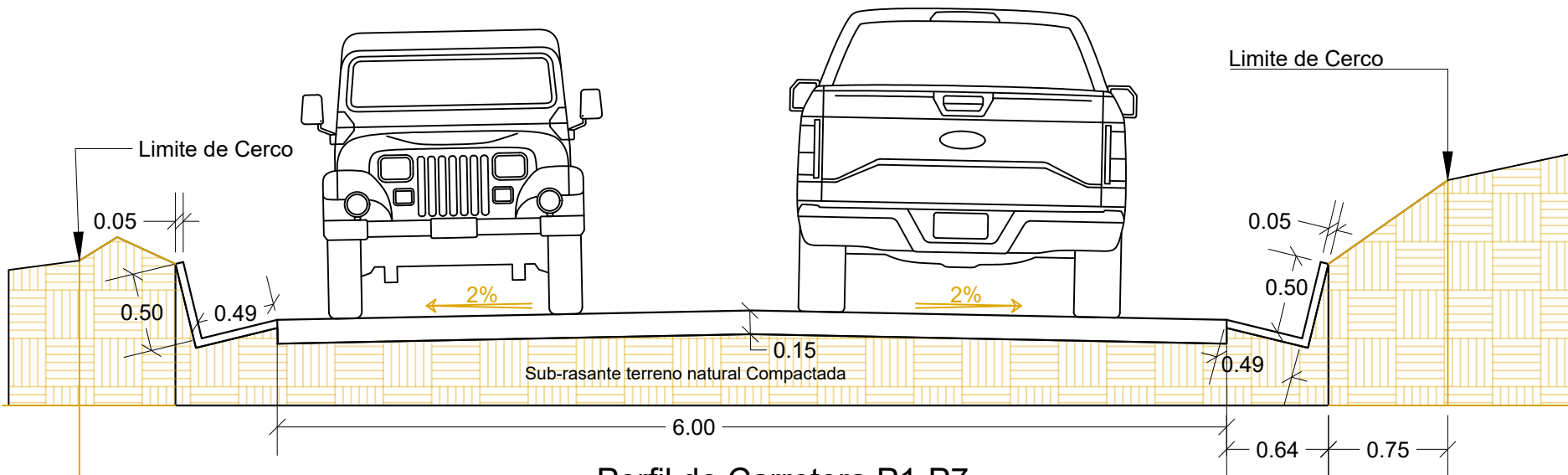
Perfil de Carretera P1-P7 Escala 1:40
