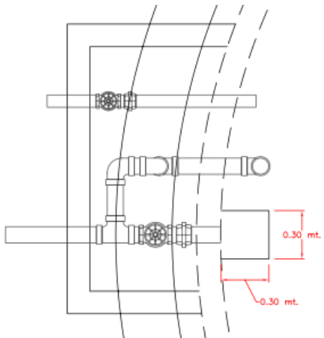
Detalle de desagüe
