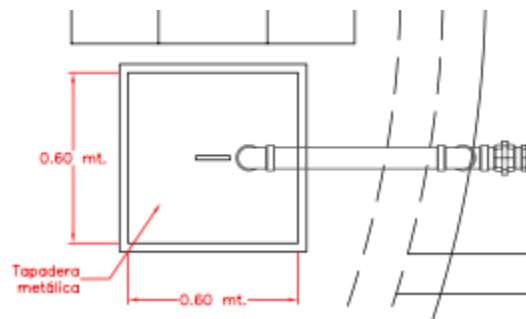
Detalle boca de inspección
