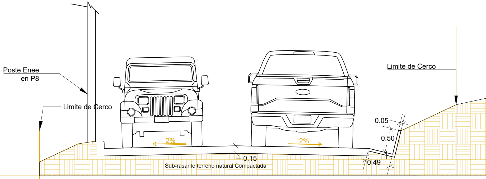
Perfil de Carretera P8-P11 Escala 1:40
