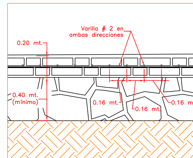
DETALLE ARMADO PISO DE LADRILLO ESCALA 1:20
