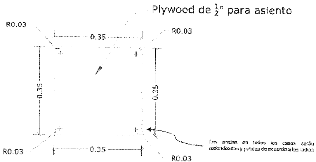
DETALLE DE ASIENTO
