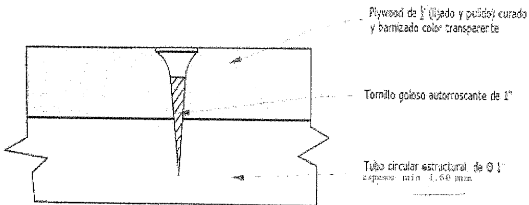
DETALLE DE ENSAMBLE DE TORNILLO SIN ESCALA
