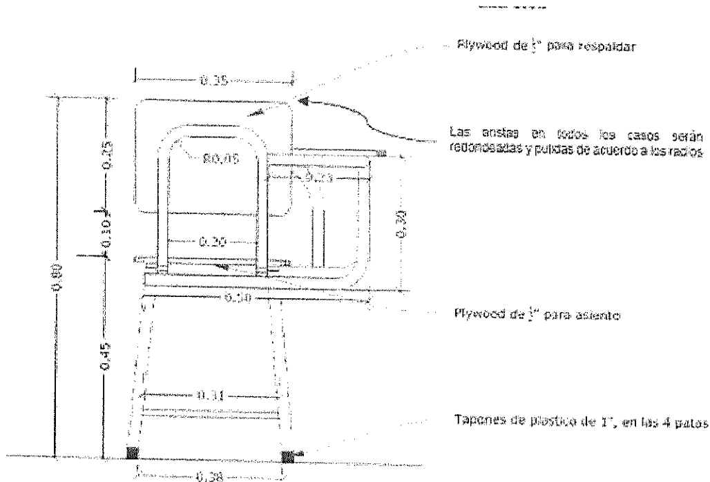
VISTA POSTERIOR DE PUPITRE ESC 1:15
