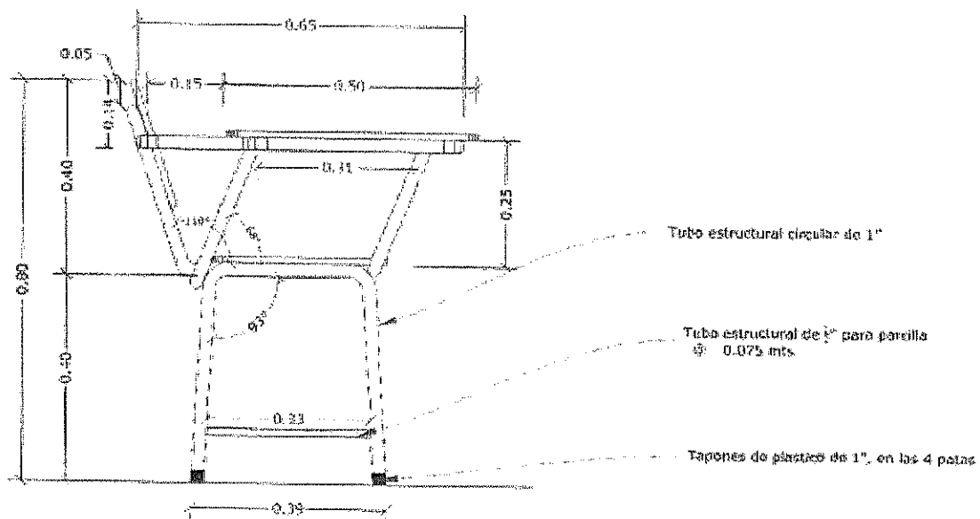
VISTA LATERAL DE PUPITRE
