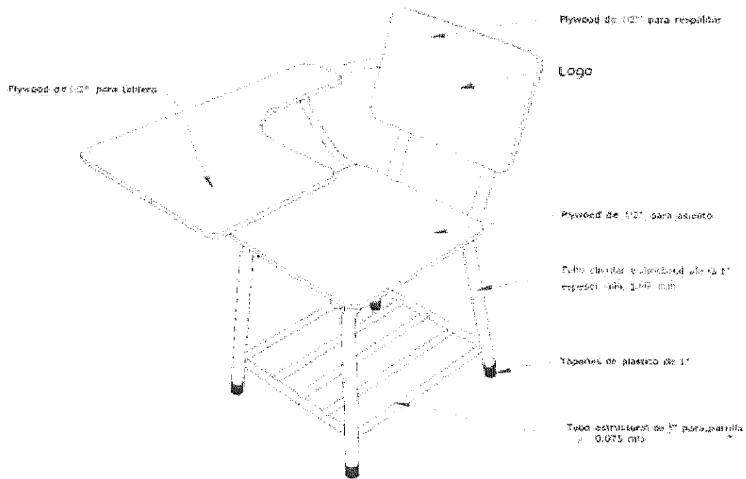
DETALLE DE PERSPECTIVA DE PUPITRE Escala: 1:1
