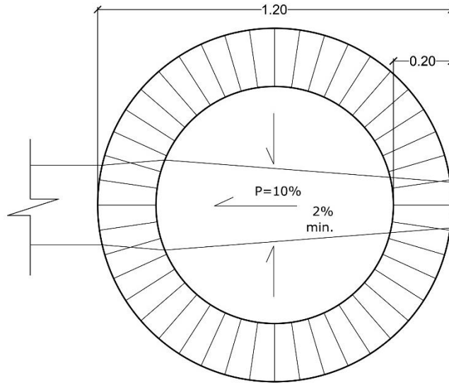
CORTE A-A
