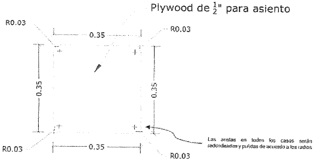
DETALLE DE ASIENTO ESC 1:10
