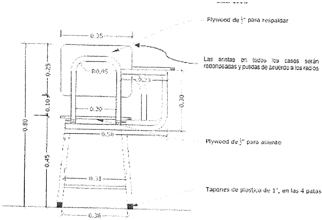
VISTA POSTERIOR DE PUPITRE ESC 1:15
