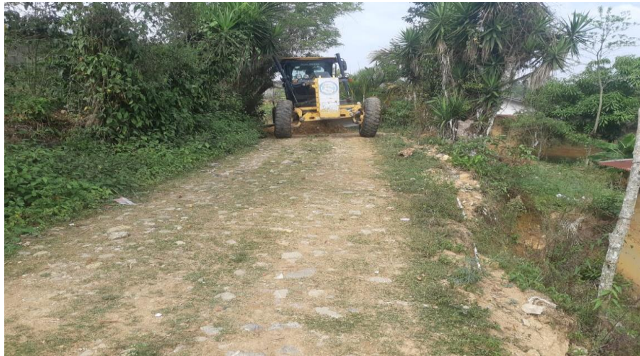
Maquina Motoniveladora 670-G y Vibro compactador en trabajos de escarificado, conformación, cuneteo y vibrado de calle que conduce hacia la aldea Cuchilla Zapa.
