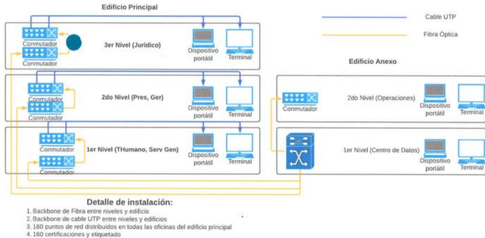
Diagrama Lógico
