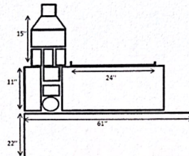
Vista Lateral
