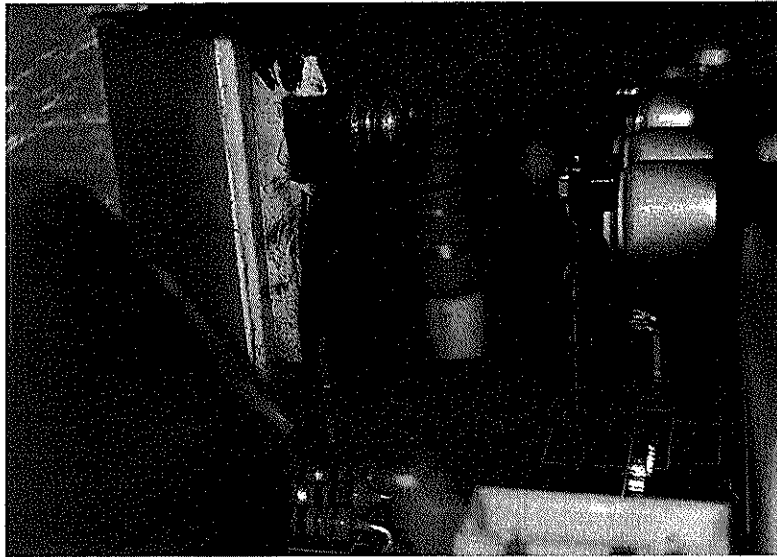
Ilustración 4 Vista del diodo de potencia reventado en la tarjeta del inversor
