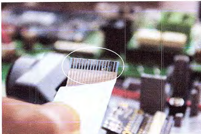
Cortocircuito en los contactos principales que comunican la placa base con el lector de huella dactilar en el cable plano flexible de circuito impreso
