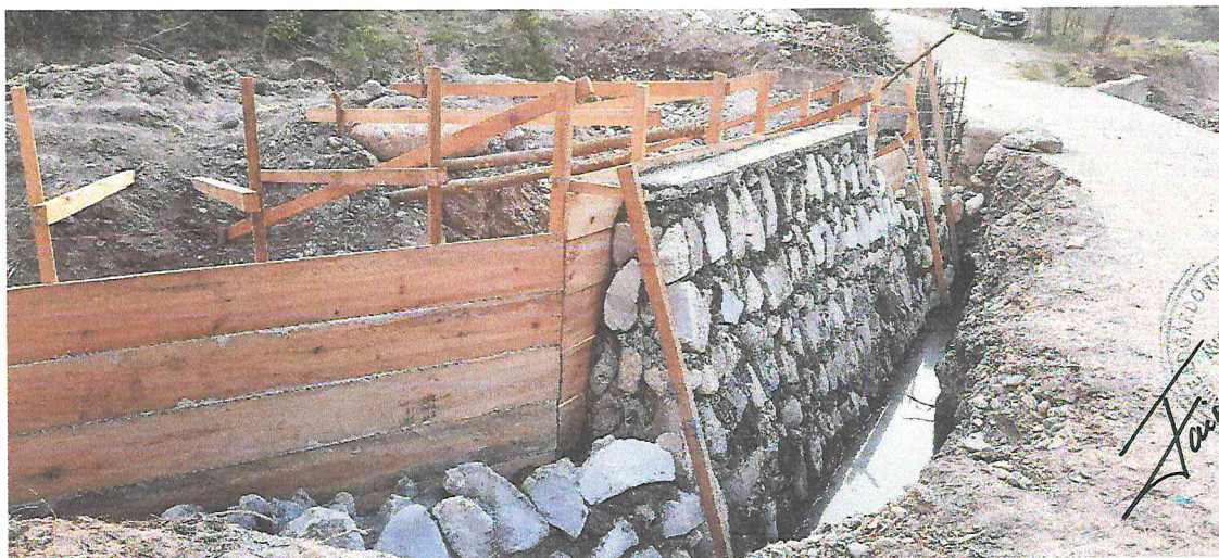
Durante la construcción del muro de contención del ala Sur-Oeste en la caja puente sobre la quebrada Saisoque.
