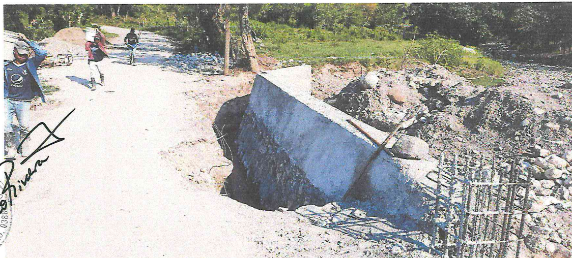
Muro del ala Sur-oeste una vez finalizado – caja puente hacia San Pablo del Roble.
