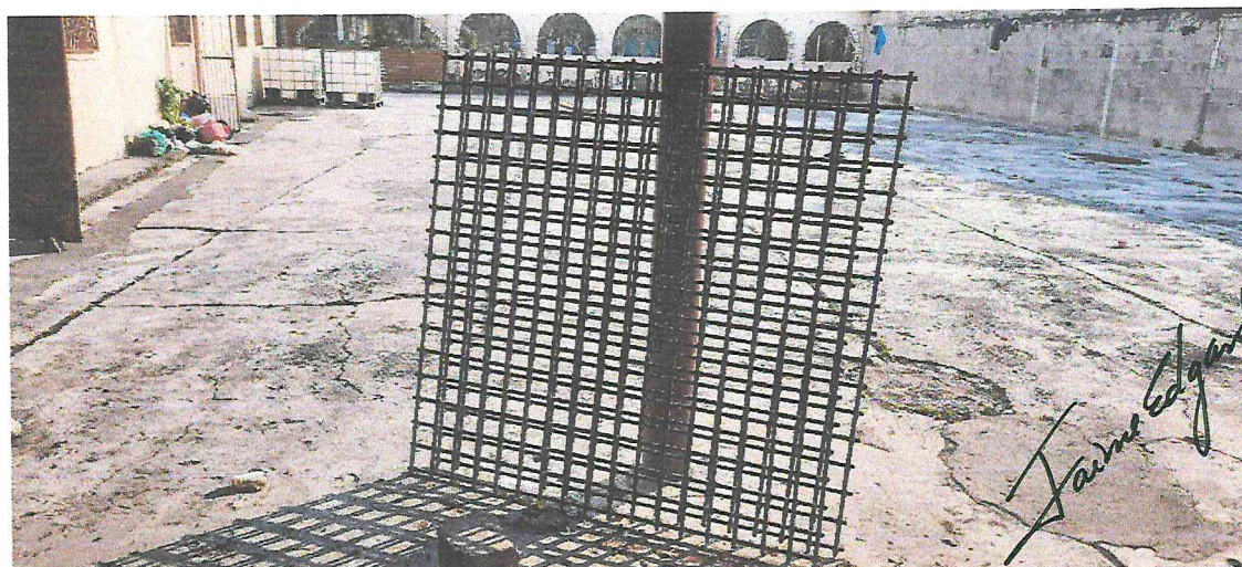
Refuerzo de doble cama para las zapatas aisladas en la subestructura de la caja puente hacia San Pablo del Roble.
