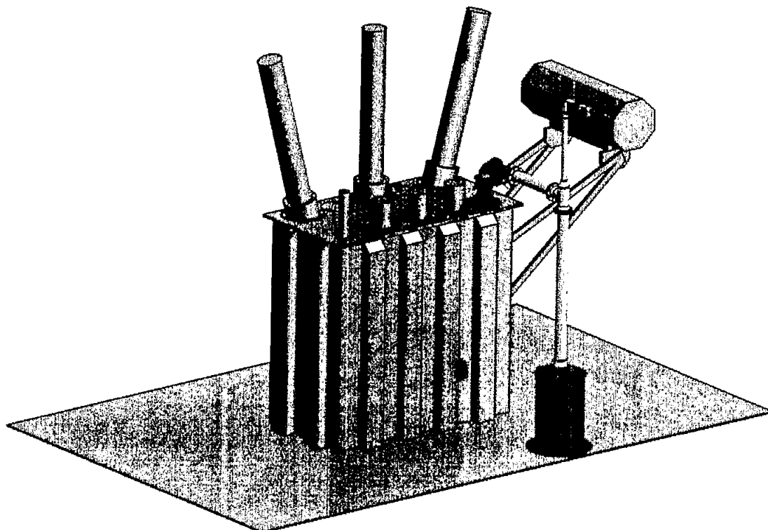
Figura 2. Segundo dibujo esquemático de un sistema de prevención de incendios y explosiones
