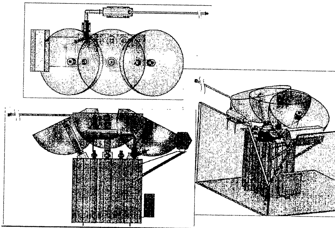
Figura 1. Dibujo esquemático de un sistema de prevención de incendios y explosiones
