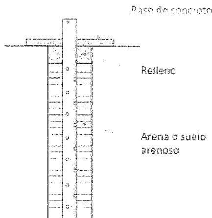
Figura 2: Ejemplo de la Especificación para tubería PVC perforada
