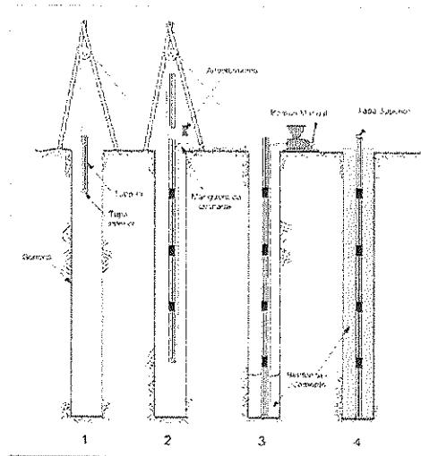
Figura 1: Ejemplo del Procedimiento para Instalación de Tubería Inclinométrica
