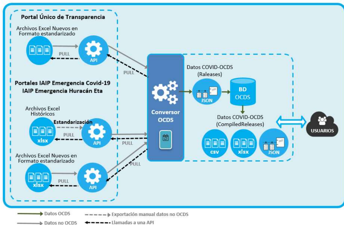
Imagen 1: Diagrama del proceso para la creación de conjuntos de datos.
